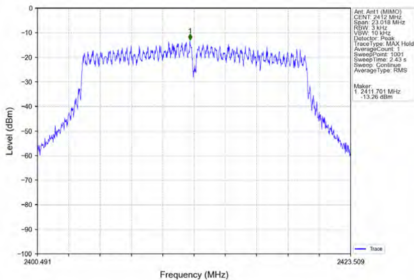
802.11g_LCH_2412MHz_Ant1 (MIMO)_NTNV
