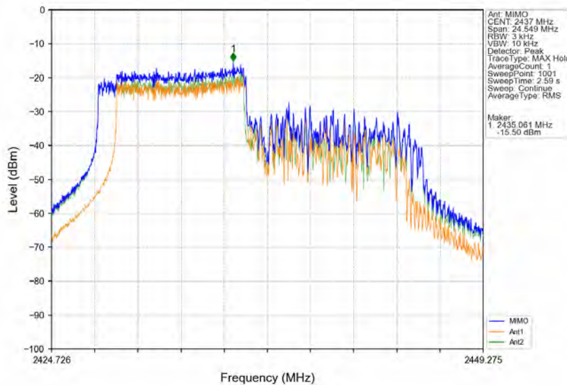
802.11ax(HE20) MCH 2437MHz RU106 Left MIMO NTN
