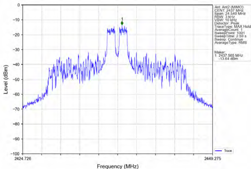
802.11ax(HE20) MCH 2437MHz RU26 Mid Ant2 (MIMO) NTVN
