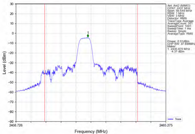
802.11ax(HE40) MCH 2437MHz RU52 Mid Ant2 (MIMO) NTVN
