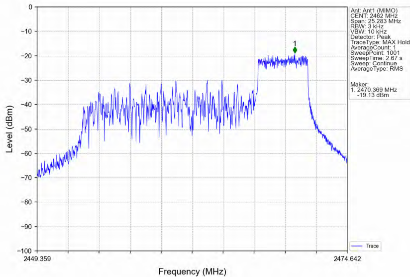
802.11ax(HE20) HCH 2462MHz RU52 Right Ant1 (MIMO) NTNv
