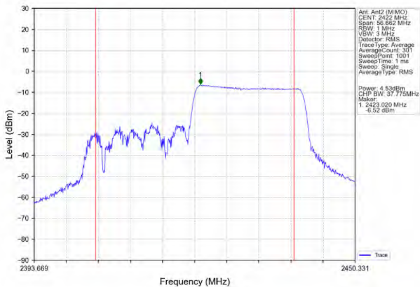
802.11ax(HE40) LCH 2422MHz RU242 Right Ant2 (MIMO) NTNW
