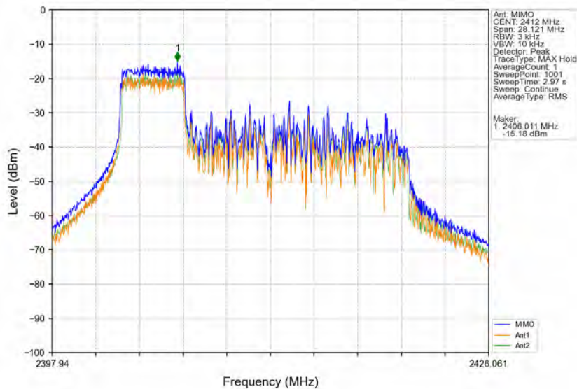
802.11ax(HE20) LCH 2412MHz RU52 Left MIMO NTN
