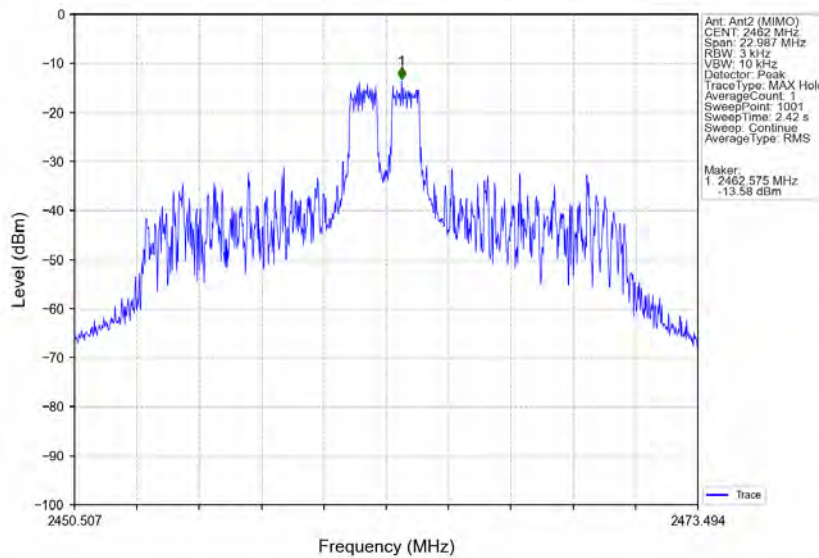
802.11ax(HE20) HCH 2462MHz RU26 Mid MIMO NTN
