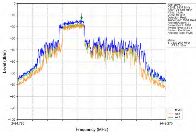
802.11ax(HE20) MCH 2437MHz RU52 Mid MIMO NTVN
