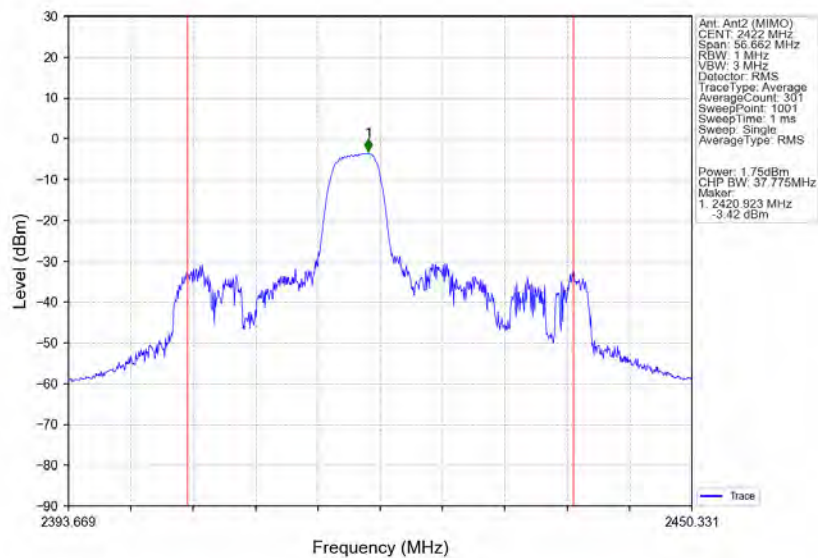
802.11ax(HE40) LCH 2422MHz RU52 Mid Ant2 (MIMO) NTVN
