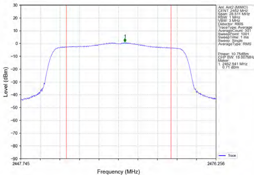
802.11ax(HE20) HCH 2462MHz RU242 Left Ant2 (MIMO) NTN
