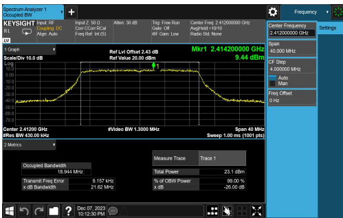
11AX20MIMO-Ant1-2412
