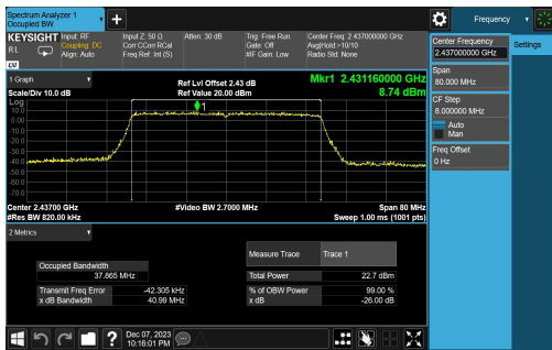
11AX40MIMO-Ant1-2437
