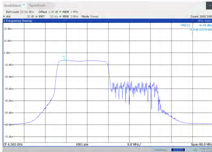
11ax40MIMO_Ant1_6565_242Tone_RU61
