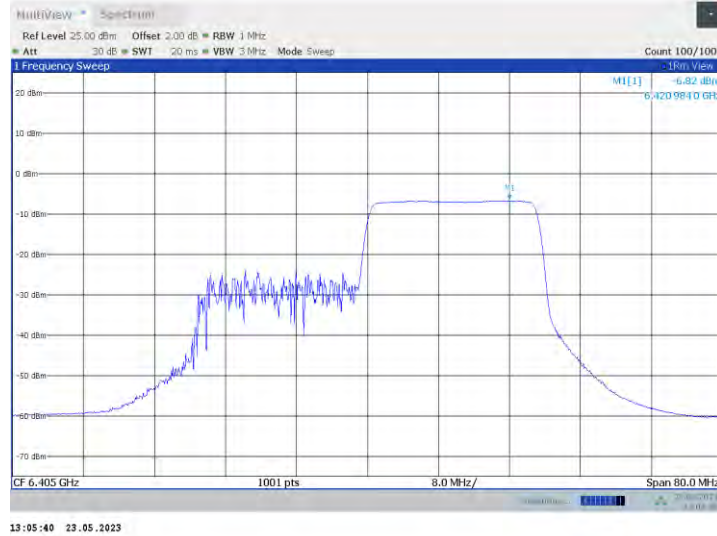
11ax40MIMO_Ant1_6405_242Tone_RU62
