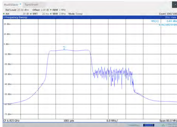
11ax40MIMO_Ant1_6925_242Tone_RU61
