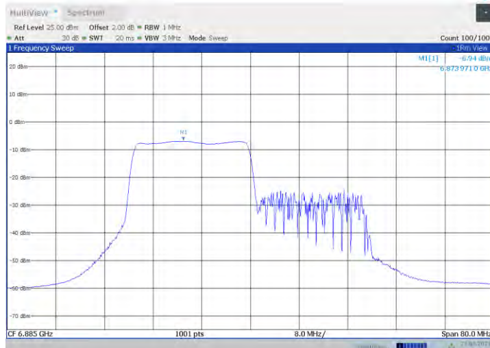
11ax40MIMO_Ant1_6885_242Tone_RU61
