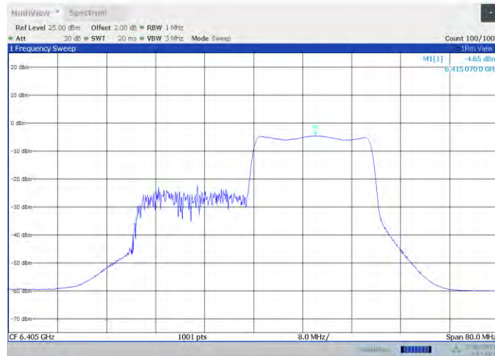
11ax40MIMO_Ant1_6405_242Tone_RU62
