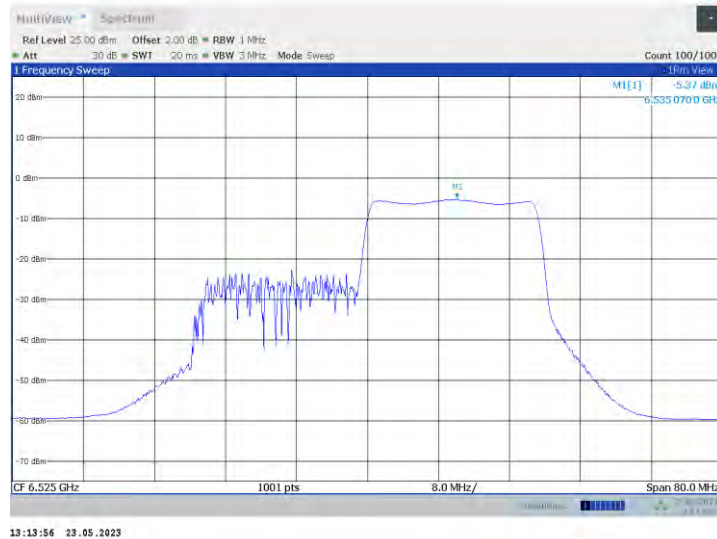
11ax40MIMO_Ant1_6525_242Tone_RU62
