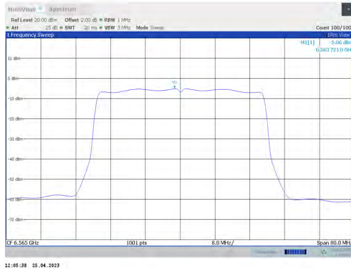
11ax40MIMO_Ant1_6565
