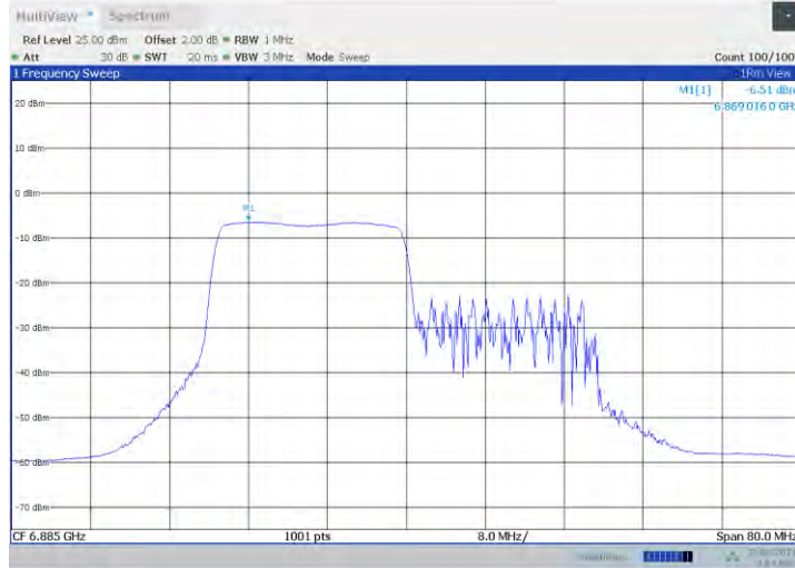
11ax40MIMO_Ant1_6885_242Tone_RU61
