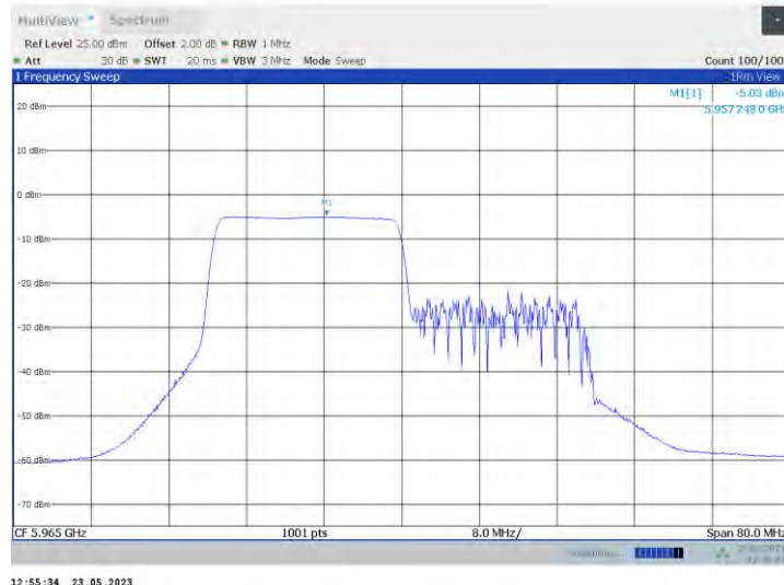
11ax40MIMO_Ant1_5965_242Tone_RU61
