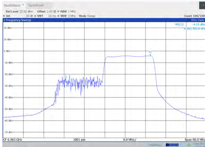
11ax40MIMO_Ant1_6965_242Tone_RU62
