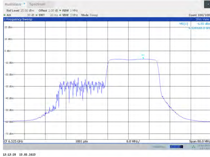
11ax40MIMO_Ant1_6525_242Tone_RU62
