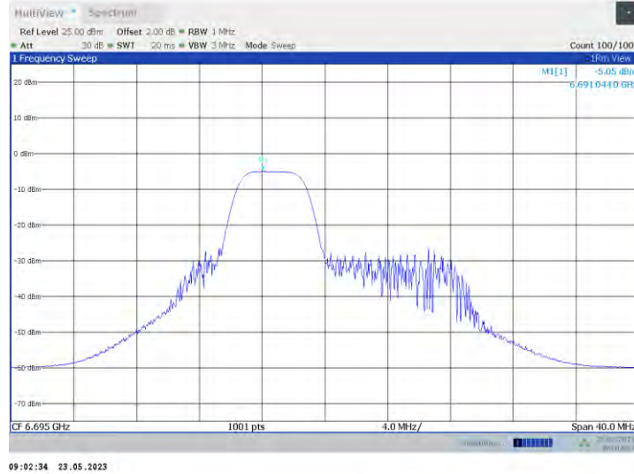
11ax20MIMO Ant1 6695 106Tone RU53
