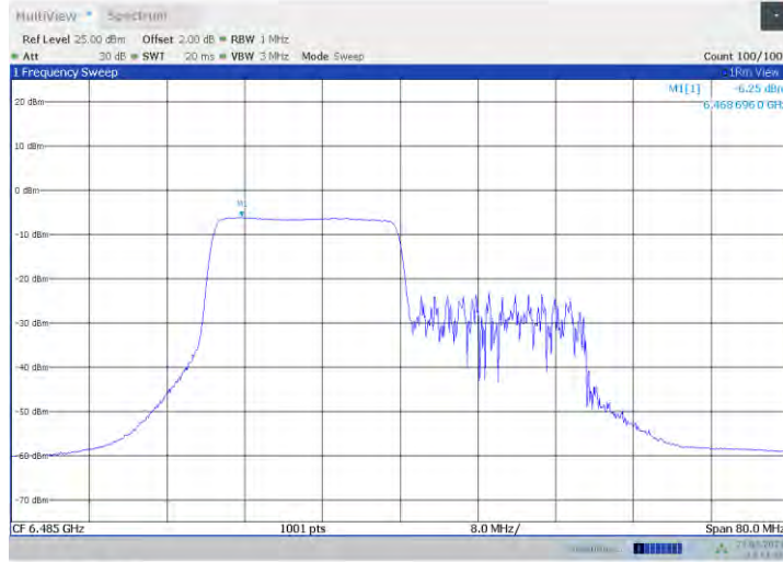
11ax40MIMO_Ant1_6485_242Tone_RU61
