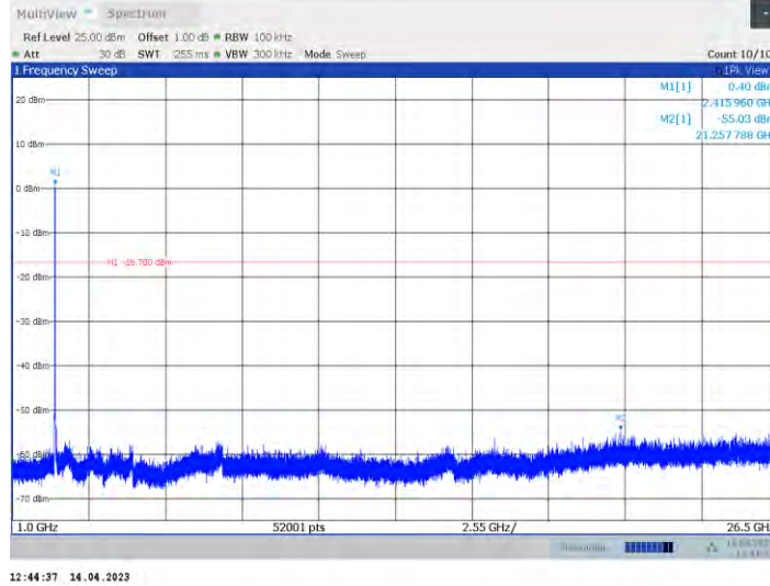
11ax20MIMO_Ant1_2412_0~Reference
