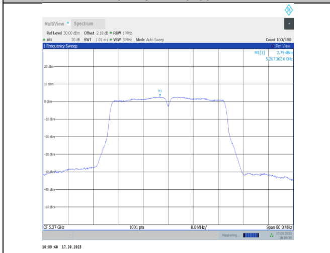
11n40SISO-Ant1-5270-PASS
