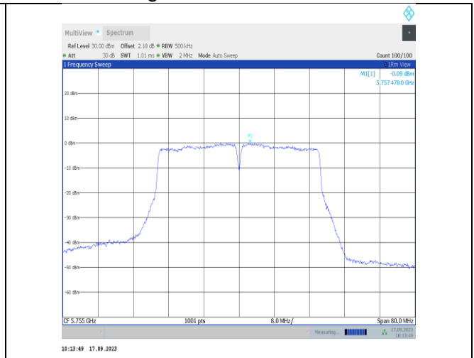
11n40SISO-Ant1-5755-PASS
