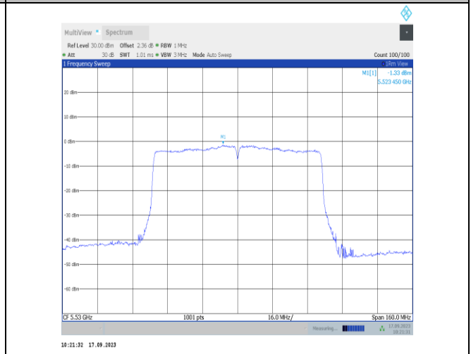
11ac80SISO-Ant1-5530-PASS
