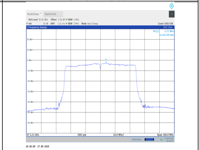
11ac80SISO-Ant1-5210-PASS
