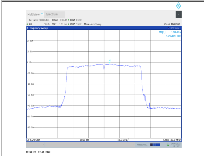
11ac80SISO-Ant1-5290-PASS
