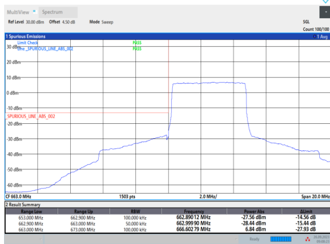
Band71-5MHz-QPSK-133147-25RB#0
