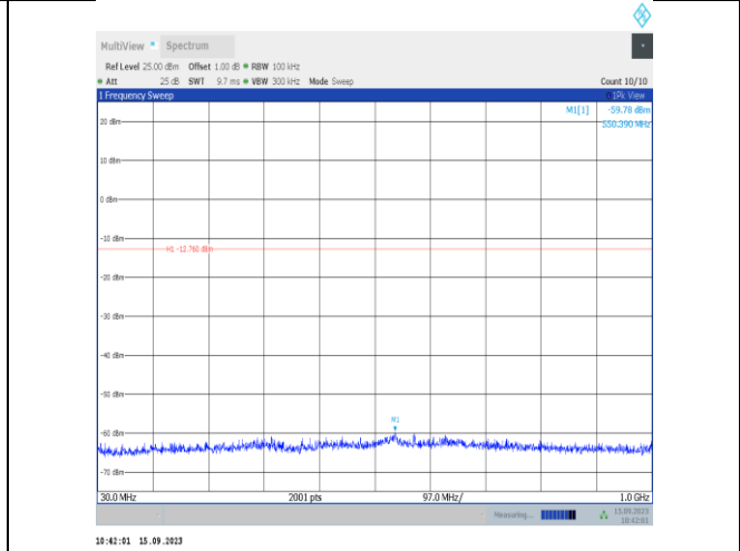
11g-Ant1-2437-30~1000-PASS
