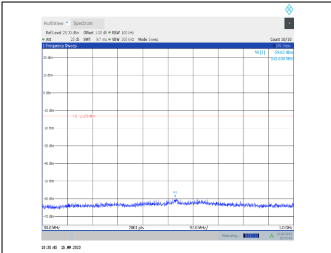
11g-Ant1-2412-30~1000-PASS
