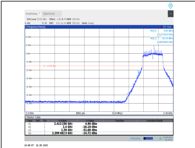
11n20ISO-Ant1-2412-PASS
