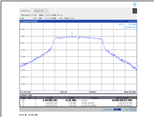
11g-Ant1-2437
