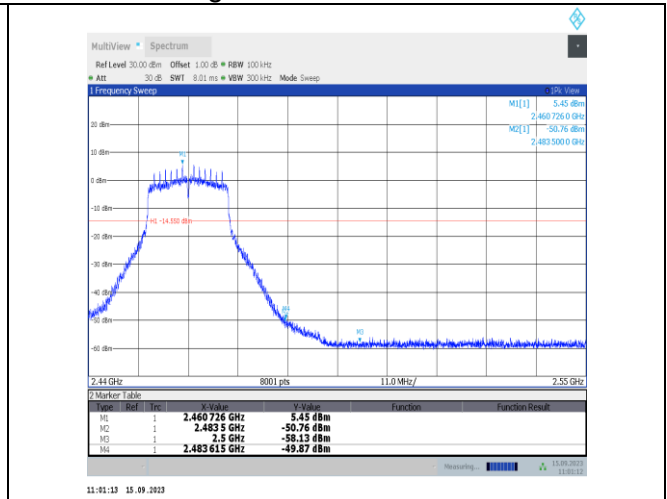
11n20ISO-Ant1-2462-PASS
