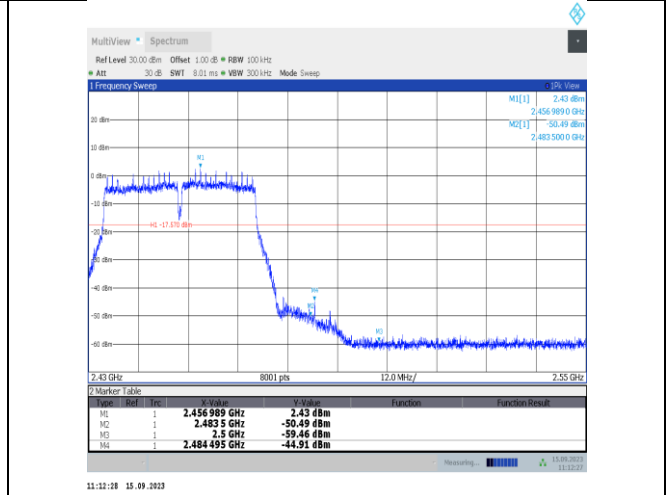
11n40ISO-Ant1-2452-PASS
