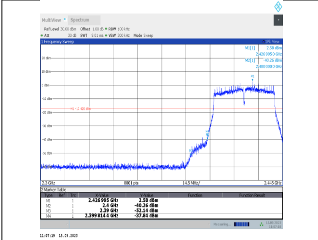
11n40ISO-Ant1-2422-PASS
