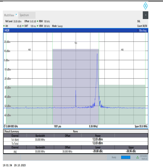
NTNV_N48_PC3_30_30_H_TID18_#1_-30_30
