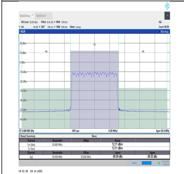
NTNV_N48_PC3_30_30_H_TID16_#1_-30_30
