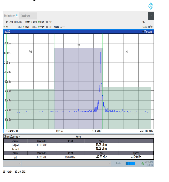
NTNV_N48_PC3_30_30_H_TID3_#1_-30_30
