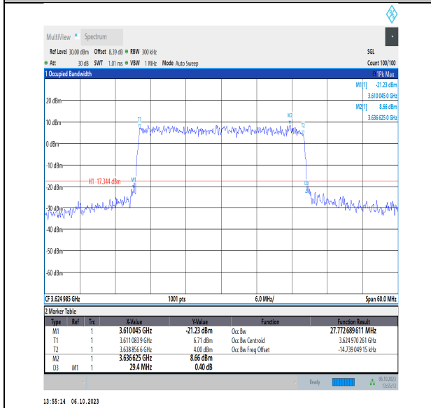
NTNV_N48_PC3_30_30_M_TID7_Ant2#1
