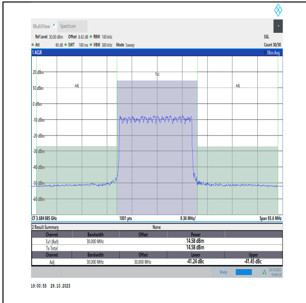
NTNV_N48_PC3_30_30_H_TID1_#1_-30_30
