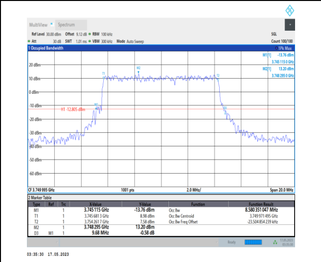
1-N78-3700-3800-PC1-30-10-M-7-CP-16QAM-Outer_Full-24@0-Ant0-8.58-9.680-≤10-PASS
