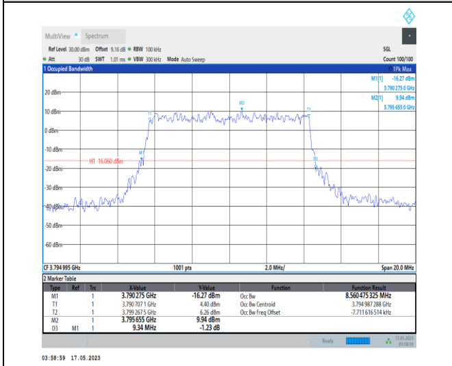
1-N78-3700-3800-PC1-30-10-H-9-CP-256QAM-Outer _Full-24@0-Ant0-8.56-9.340-≤10-PASS
