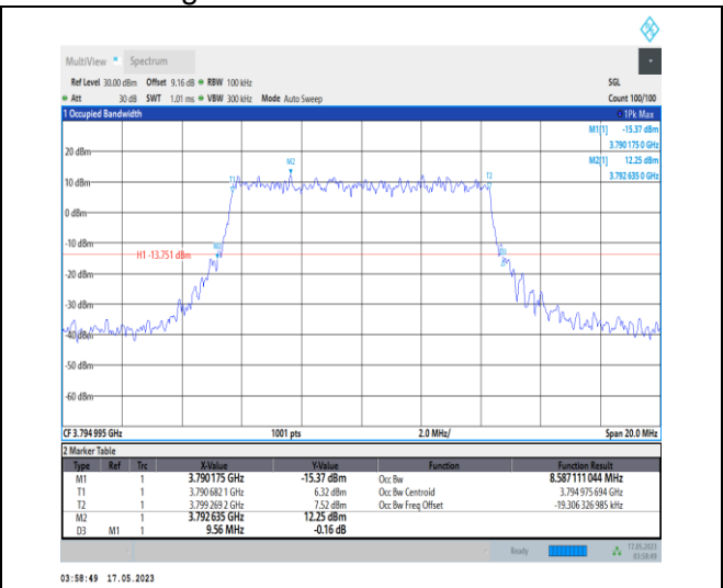
1-N78-3700-3800-PC1-30-10-H-8-CP-64QAM-Outer _Full-24@0-Ant0-8.587-9.560-≤10-PASS
