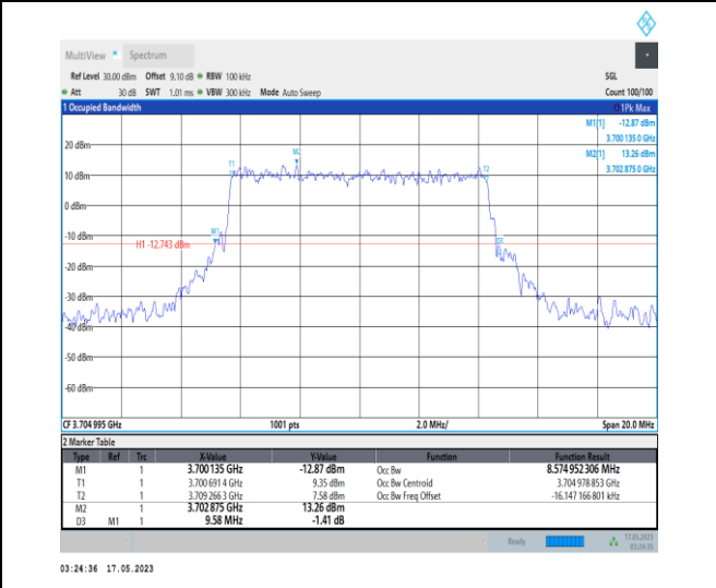
1-N78-3700-3800-PC1-30-10-L-8-CP-64QAM-Outer _Full-24@0-Ant0-8.575-9.580-≤10-PASS
