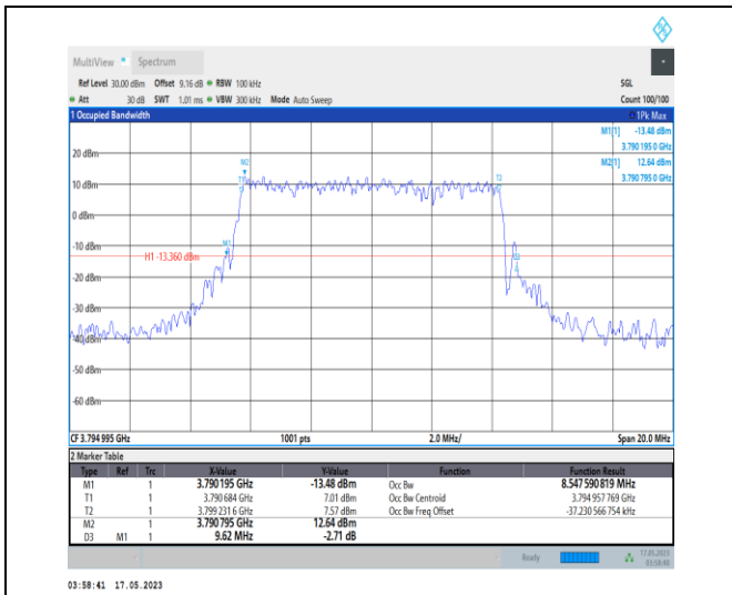
1-N78-3700-3800-PC1-30-10-H-7-CP-16QAM-Outer _Full-24@0-Ant0-8.548-9.620-≤10-PASS
