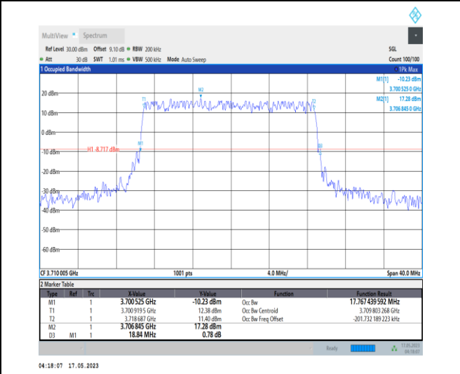
1-N78-3700-3800-PC1-30-20-L-2-DFT-PI2BPSK-Outer_Full-50@0-Ant0-17.767-18.840-≤20-PASS
