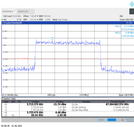
1-N78-3700-3800--30-70-M-9-CP-256QAM-Outer_F ull-189@0-Ant0-67.505-69.440-≤70-PASS
