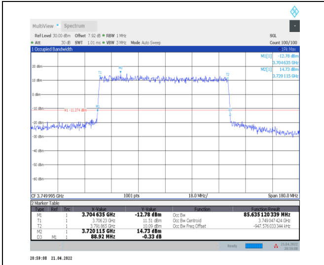
1-N78-3700-3800--30-90-M-1-DFT-QPSK-Outer_Full -240@0-Ant0-85.635-88.920-≤90-PASS
