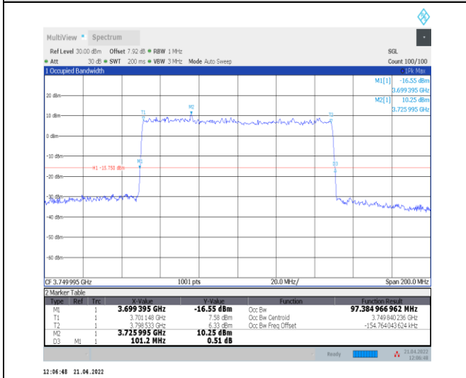
1-N78-3700-3800--30-100-L-9-CP-256QAM-Outer_Fu II-273@0-Ant0-97.385-101.200-≤100-PASS
