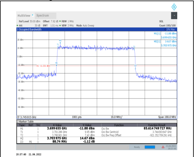
1-N78-3700-3800--30-90-L-3-DFT-16QAM-Outer_Fu ll-240@0-Ant0-85.615-88.740-<math>\leq 90</math>-PASS
