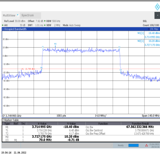
1-N78-3700-3800--30-70-M-7-CP-16QAM-Outer_Full -189@0-Ant0-67.562-70.000-≤70-PASS
