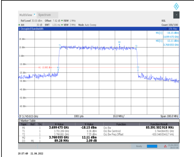
1-N78-3700-3800--30-90-L-4-DFT-64QAM-Outer_Ful l-240@0-Ant0-85.592-89.280-<math>\leq 90</math>-PASS
