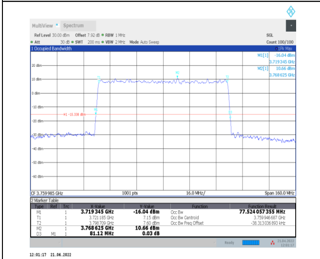
1-N78-3700-3800--30-80-H-9-CP-256QAM-Outer_Fu ll-217@0-Ant0-77.524-81.120-≤80-PASS
