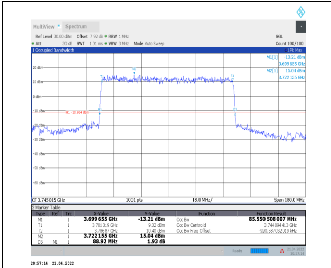
1-N78-3700-3800--30-90-L-2-DFT-PI2BPSK-Outer_F ull-240@0-Ant0-85.551-88.920-<math>\leq 90</math>-PASS
