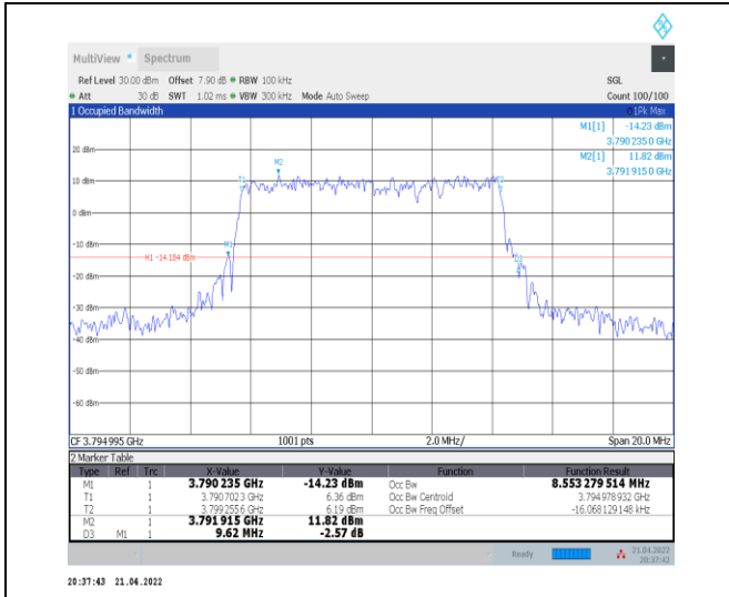
1-N78-3700-3800--30-10-H-3-DFT-16QAM-Outer_Fu II-24@0-Ant0-8.553-9.620-≤10-PASS
