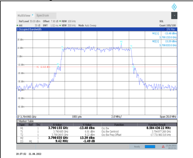
1-N78-3700-3800--30-10-H-4-DFT-64QAM-Outer_Fu II-24@0-Ant0-8.584-9.420-≤10-PASS
