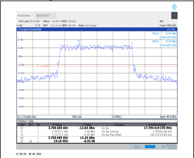
1-N78-3700-3800--30-20-L-4-DFT-64QAM-Outer_Fu II-50@0-Ant0-17.794-19.160-<math>\leq 20</math>-PASS
