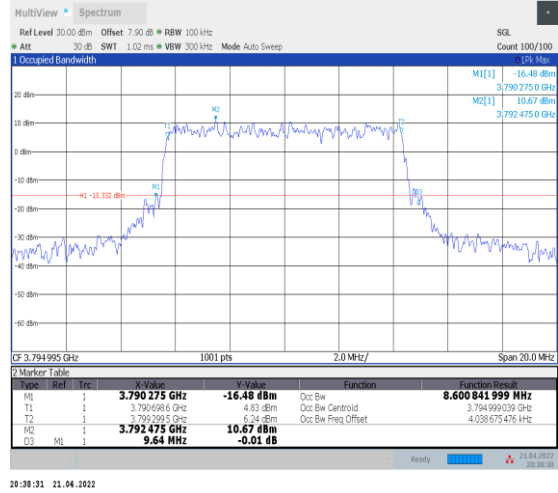
1-N78-3700-3800--30-10-H-8-CP-64QAM-Outer_Full -24@0-Ant0-8.601-9.640≤10-PASS
