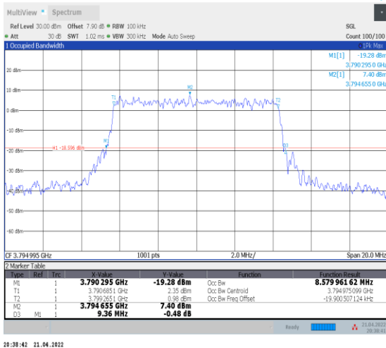
1-N78-3700-3800--30-10-H-9-CP-256QAM-Outer_Fu ll-24@0-Ant0-8.58-9.360≤10-PASS
