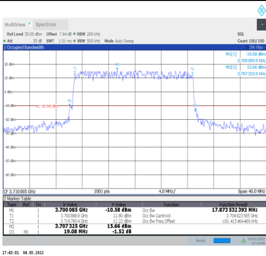
1-N78-3700-3800--30-20-L-1-DFT-QPSK-Outer_Full 50@0-Ant0-17.874-19.080-≤20-PASS
