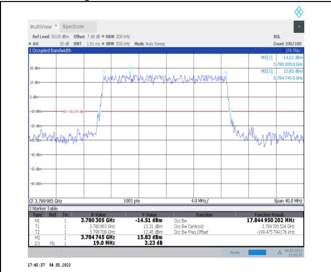
1-N78-3700-3800--30-20-H-2-DFT-PI2BPSK-Outer_Full -50@0-Ant0-17.845-19.000-≤20-PASS
