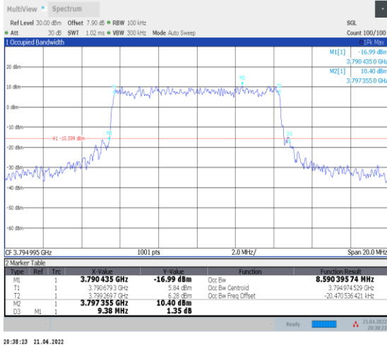
1-N78-3700-3800--30-10-H-7-CP-16QAM-Outer_Full -24@0-Ant0-8.59-9.380≤10-PASS
