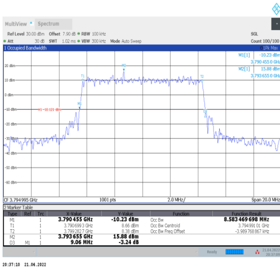
1-N78-3700-3800--30-10-H-1-DFT-QPSK-Outer_Full -24@0-Ant0-8.583-9.060-≤10-PASS
