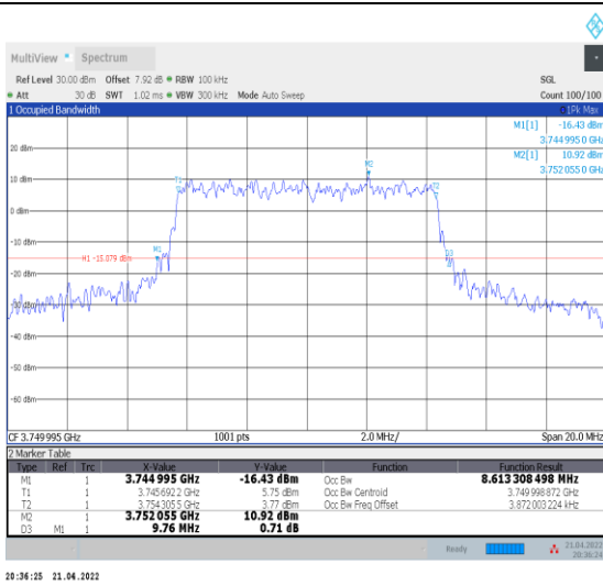
1-N78-3700-3800--30-10-M-8-CP-64QAM-Outer_Full -24@0-Ant0-8.613-9.760-≤10-PASS
