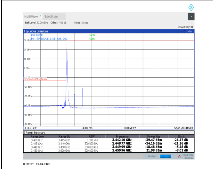
1-N78-3450-3550--30-20-L-4-CP-QPSK-Edge_1RB_L eft-1@0-Ant0-PASS-see graph
