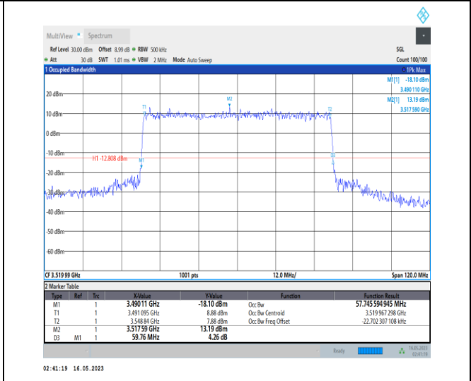
1-N78-3450-3550-PC1-30-60-H-8-CP-64QAM-Outer _Full-162@0-Ant0-57.746-59.760-≤60-PASS
