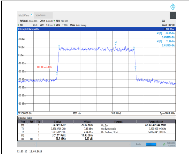
1-N78-3450-3550-PC1-30-50-M-9-CP-256QAM-Out er_Full-133@0-Ant0-47.369-49.700-≤50-PASS
