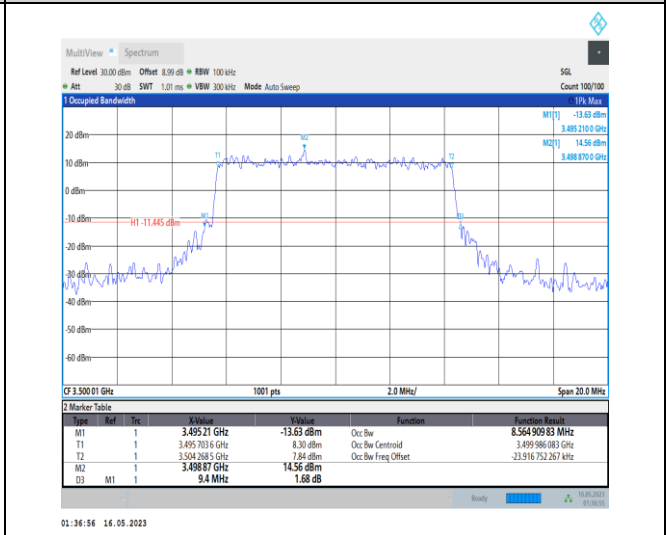
1-N78-3450-3550-PC1-30-10-M-7-CP-16QAM-Outer_Full-24@0-Ant0-8.565-9.400-≤10-PASS
