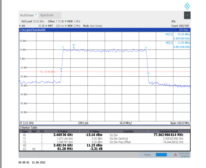
1-N78-3450-3550--30-80-H-9-CP-256QAM-Outer_Fu ll-217@0-Ant0-77.563-81.280≤80-PASS
