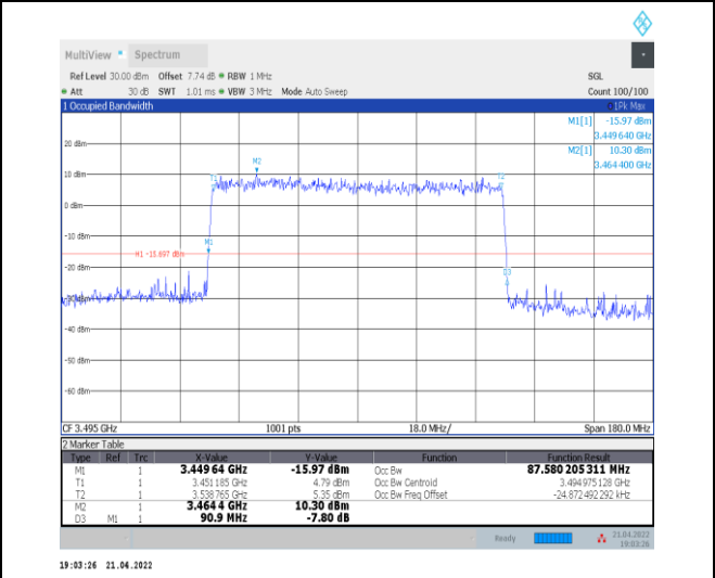
1-N78-3450-3550--30-90-L-9-CP-256QAM-Outer_Fu II-245@0-Ant0-87.58-90.900≤90-PASS
