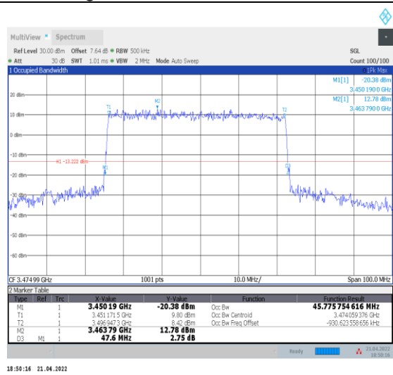
1-N78-3450-3550--30-50-L-3-DFT-16QAM-Outer_Fu ll-128@0-Ant0-45.776-47.600-≤50-PASS
