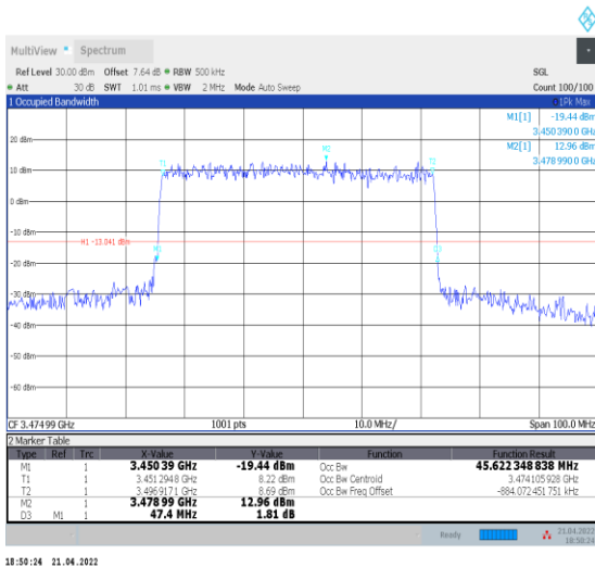
1-N78-3450-3550--30-50-L-4-DFT-64QAM-Outer_Ful l-128@0-Ant0-45.622-47.400-≤50-PASS
