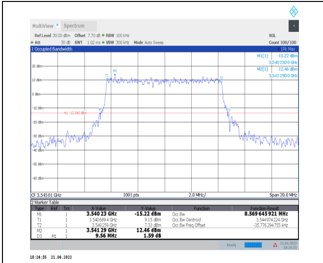
1-N78-3450-3550--30-10-H-3-DFT-16QAM-Outer_Fu II-24@0-Ant0-8.57-9.560-≤10-PASS
