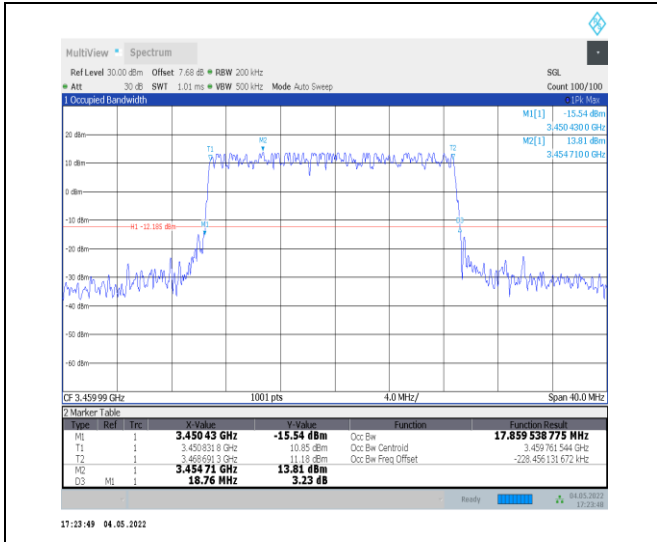
1-N78-3450-3550--30-20-L-3-DFT-16QAM-Outer_Ful I-50@0-Ant0-17.86-18.760-<=20-PASS
