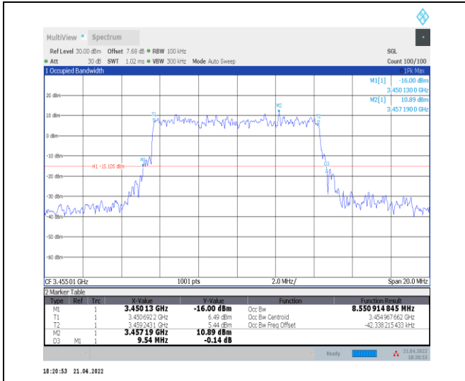
1-N78-3450-3550--30-10-L-5-DFT-256QAM-Outer_Full-24@0-Ant0-8.551-9.540-≤10-PASS
