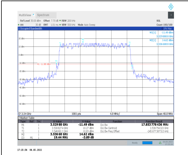
1-N78-3450-3550--30-20-H-1-DFT-QPSK-Outer_Full -50@0-Ant0-17.854-19.440-≤20-PASS
