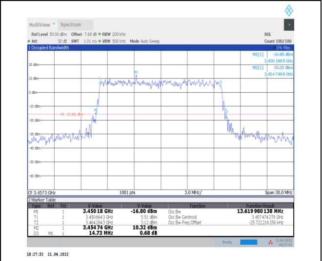
1-N78-3450-3550--30-15-L-9-CP-256QAM-Outer_Fu ll-38@0-Ant0-13.62-14.730-≤15-PASS
