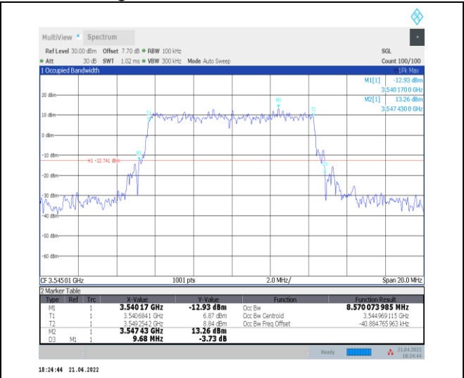
1-N78-3450-3550--30-10-H-4-DFT-64QAM-Outer_Fu II-24@0-Ant0-8.57-9.680-≤10-PASS
