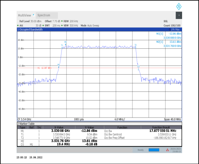
1-N78-3450-3550--30-20-H-4-DFT-64QAM-Outer_Fu II-50@0-Ant0-17.878-19.400-≤20-PASS
