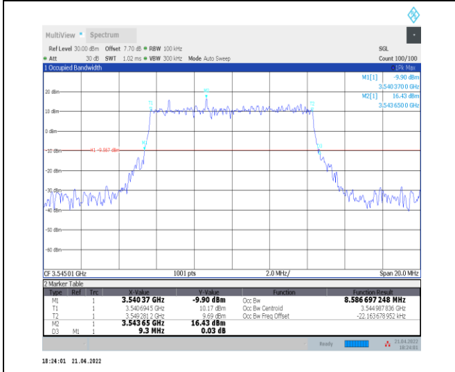
1-N78-3450-3550--30-10-H-1-DFT-QPSK-Outer_Full -24@0-Ant0-8.587-9.300-≤10-PASS
