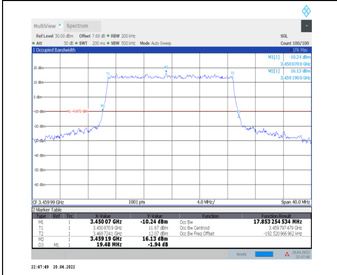
1-N78-3450-3550--30-20-L-1-DFT-QPSK-Outer_Full -50@0-Ant0-17.853-19.480-≤20-PASS
