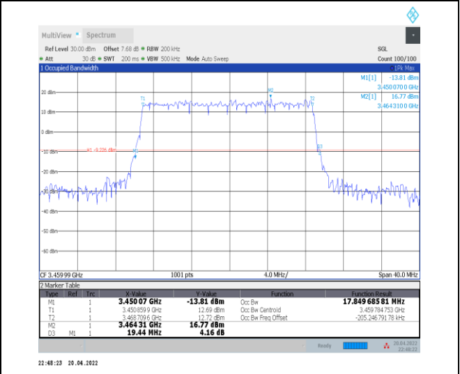
1-N78-3450-3550--30-20-L-2-DFT-PI2BPSK-Outer_Full -50@0-Ant0-17.85-19.440-≤20-PASS
