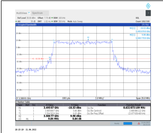
1-N78-3450-3550--30-10-M-8-CP-64QAM-Outer_Full -24@0-Ant0-8.633-9.840-≤10-PASS
