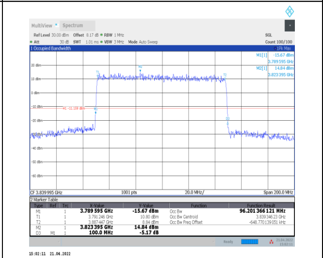
1-N77-3700-3980--30-100-M-1-DFT-QPSK-Outer_Fu I1-270@0-Ant0-96.201-100.000-≤100-PASS
