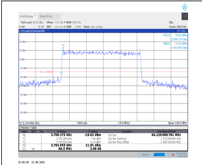
1-N77-3700-3980--30-70-L-4-DFT-64QAM-Outer_Fu II-180@0-Ant0-64.22-66.500-<math>\leq</math>70-PASS
