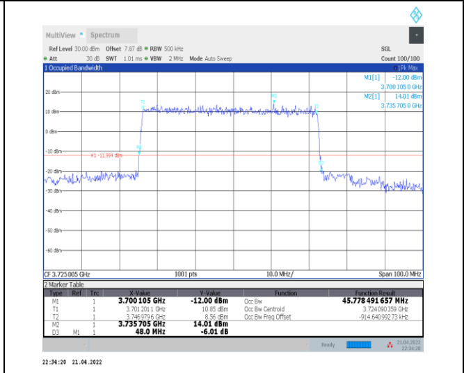
1-N77-3700-3980--30-50-L-1-DFT-QPSK-Outer_Full-128@0-Ant0-45.778-48.000-<math>\leq 50</math>-PASS
