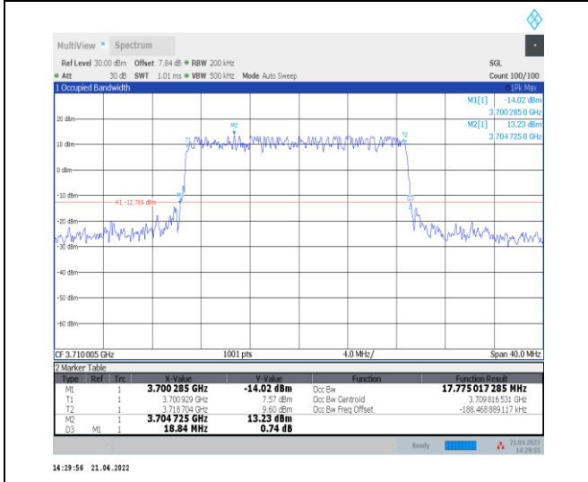
1-N77-3700-3980--30-20-L-1-DFT-QPSK-Outer_Full -50@0-Ant0-17.775-18.840≤20-PASS
