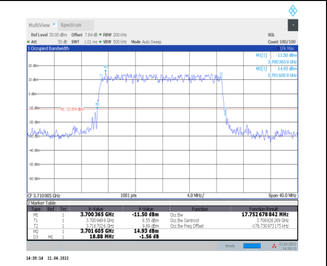
1-N77-3700-3980--30-20-L-2-DFT-PI2BPSK-Outer_Full -50@0-Ant0-17.753-18.880≤20-PASS
