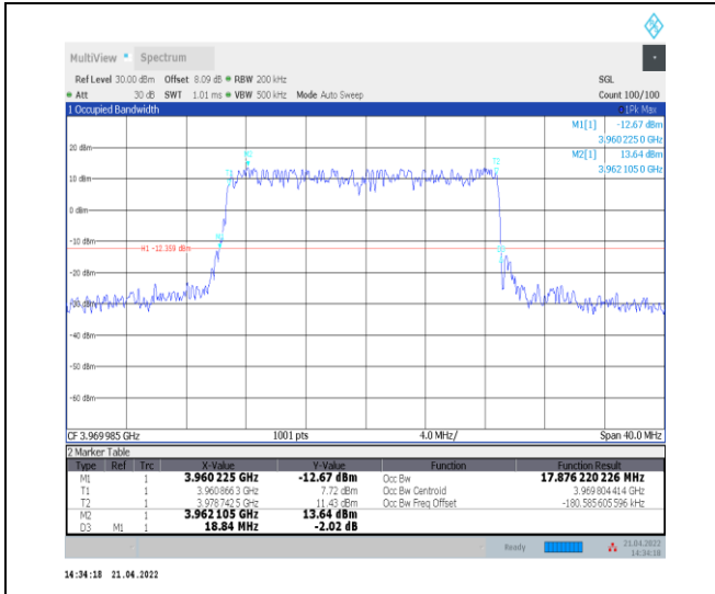
1-N77-3700-3980--30-20-H-1-DFT-QPSK-Outer_Full -50@0-Ant0-17.876-18.840-≤20-PASS
