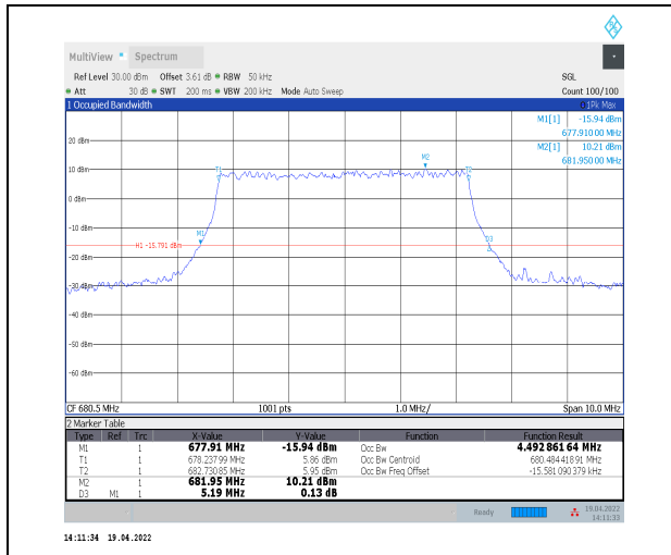
1-N71--15-5-M-8-CP-64QAM-Outer_Full-25@0-Ant0 -4.493-5.190≤5-PASS
