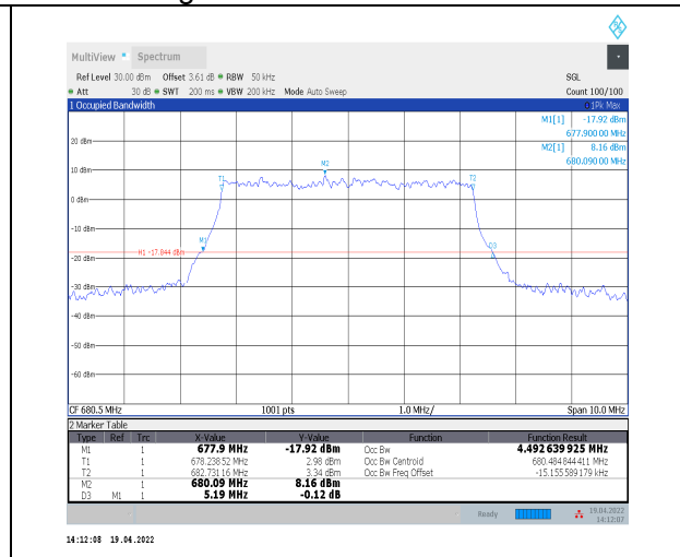
1-N71--15-5-M-9-CP-256QAM-Outer_Full-25@0-Ant 0-4.493-5.190≤5-PASS
