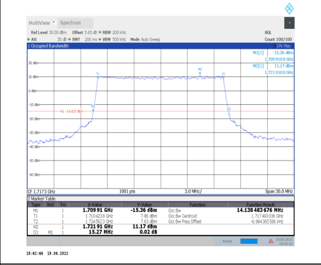
1-N66-PC3-15-15-L-6-CP-QPSK-Outer_Full-79@0-A nt0-14.138-15.270-≤15-PASS
