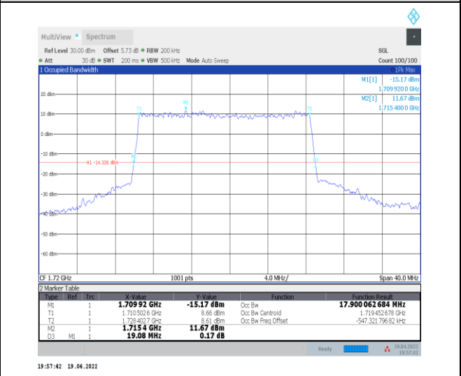
1-N66-PC3-15-20-L-3-DFT-16QAM-Outer_Full-100 @0-Ant0-17.9-19.080-≤20-PASS
