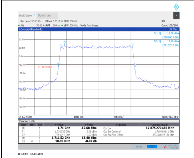
1-N66-PC3-15-20-L-2-DFT-PI2BPSK-Outer_Full-100 @0-Ant0-17.875-18.960-≤20-PASS
