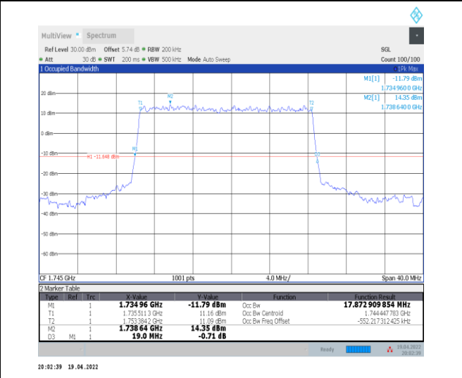
1-N66-PC3-15-20-M-2-DFT-PI2BPSK-Outer_Full-100 @0-Ant0-17.873-19.000-≤20-PASS
