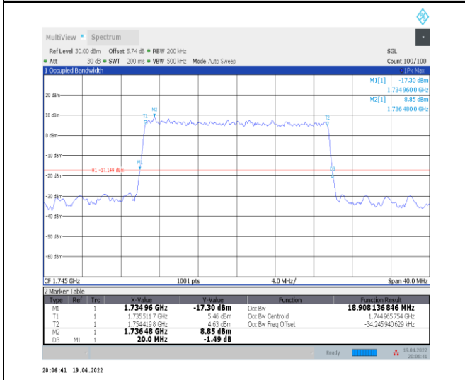
1-N66-PC3-15-20-M-9-CP-256QAM-Outer_Full-106 @0-Ant0-18.908-20.000-≤20-PASS
