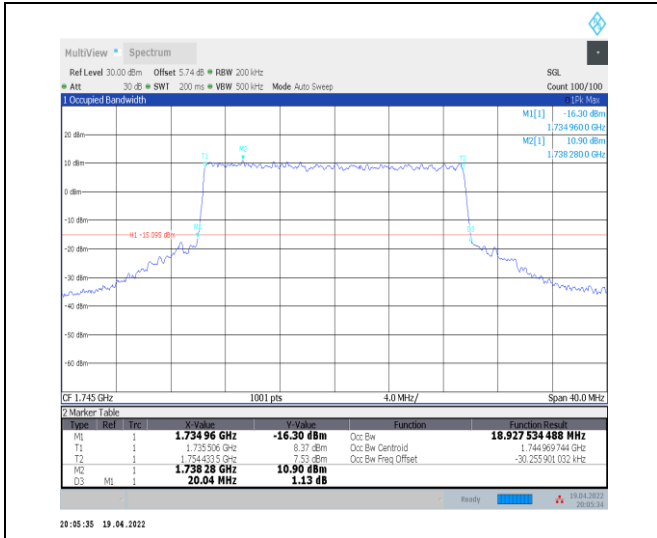
1-N66-PC3-15-20-M-7-CP-16QAM-Outer_Full-106@ 0-Ant0-18.928-20.040-≤20-PASS
