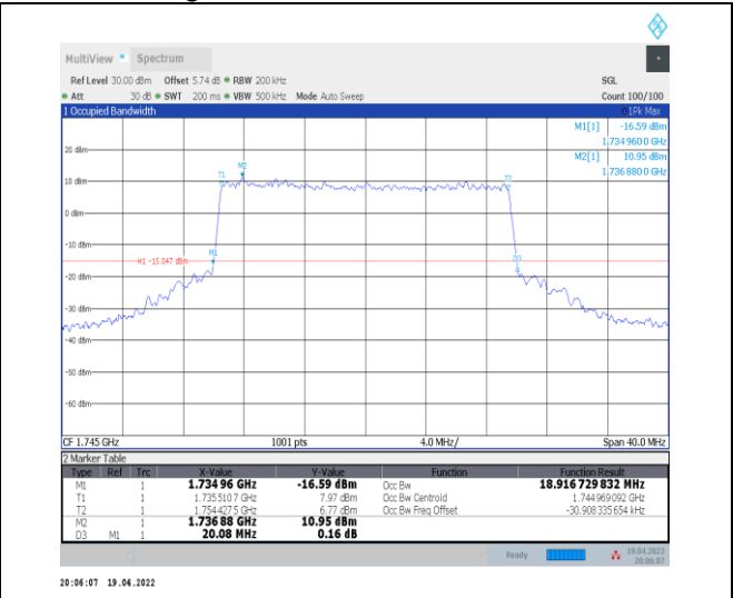
1-N66-PC3-15-20-M-8-CP-64QAM-Outer_Full-106@ 0-Ant0-18.917-20.080-≤20-PASS
