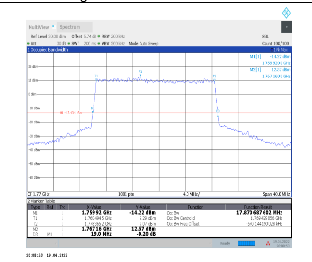
1-N66-PC3-15-20-H-3-DFT-16QAM-Outer_Full-100 @0-Ant0-17.871-19.000-≤20-PASS
