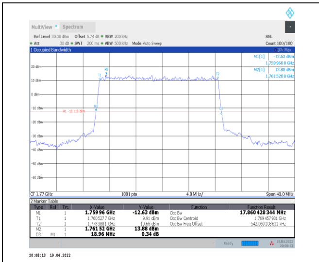
1-N66-PC3-15-20-H-2-DFT-PI2BPSK-Outer_Full-100 @0-Ant0-17.86-18.960-≤20-PASS
