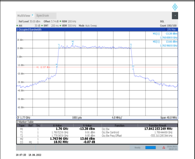
1-N66-PC3-15-20-H-1-DFT-QPSK-Outer_Full-100@ 0-Ant0-17.842-18.920-≤20-PASS
