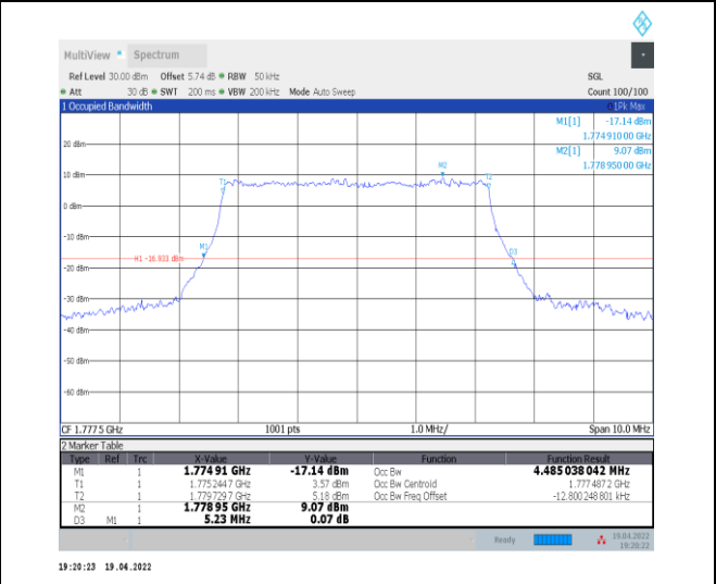
1-N66-PC3-15-5-H-6-CP-QPSK-Outer_Full-25@0-A nt0-4.485-5.230-≤5-PASS
