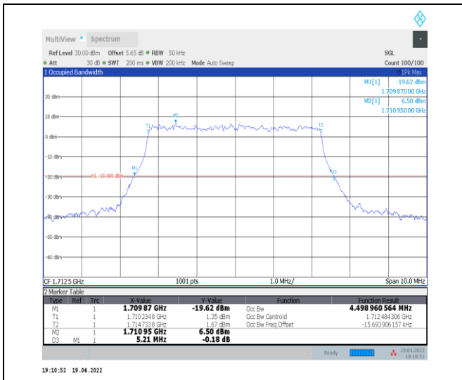
1-N66-PC3-15-5-L-9-CP-256QAM-Outer_Full-25@0-Ant0-4.499-5.210-≤5-PASS
