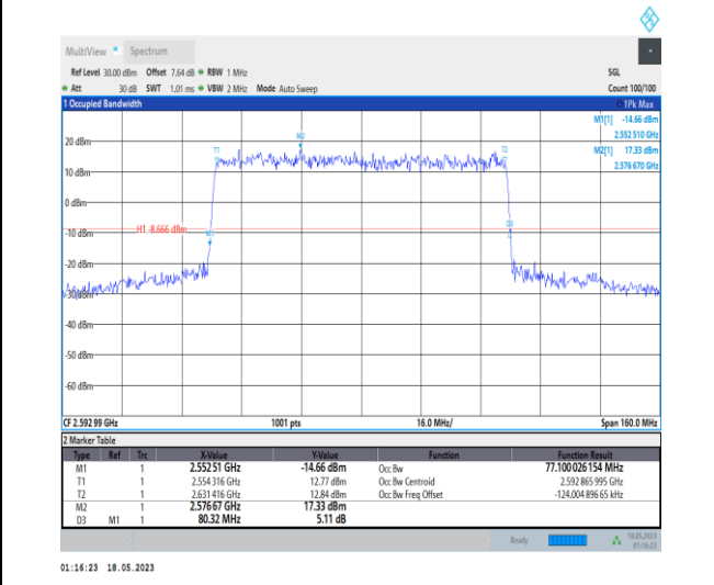
1-N41-PC1-30-80-M-1-DFT-QPSK-Outer_Full-216@ 0-Ant0-77.1-80.320-≤80-PASS
