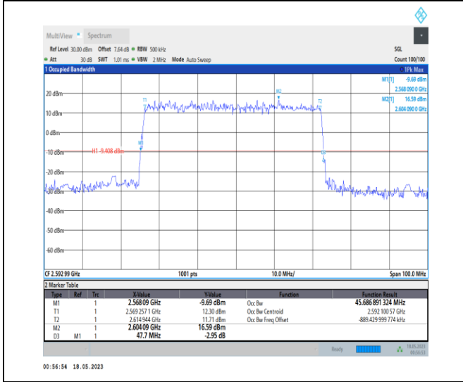
1-N41-PC1-30-50-M-1-DFT-QPSK-Outer_Full-128@ 0-Ant0-45.687-47.700-≤50-PASS
