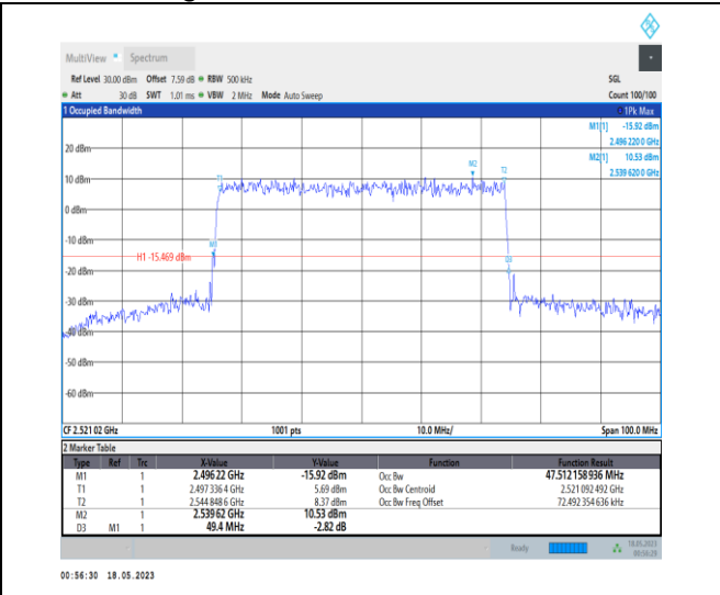
1-N41-PC1-30-50-L-9-CP-256QAM-Outer_Full-133 @0-Ant0-47.512-49.400-≤50-PASS
