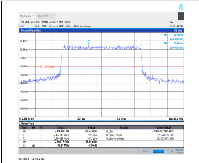
1-N41-PC1-30-40-L-7-CP-16QAM-Outer_Full-106@ 0-Ant0-37.838-39.840-≤40-PASS
