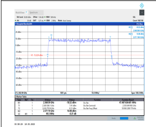
1-N41-PC1-30-50-M-9-CP-256QAM-Outer_Full-133 @0-Ant0-47.488-49.500-≤50-PASS
