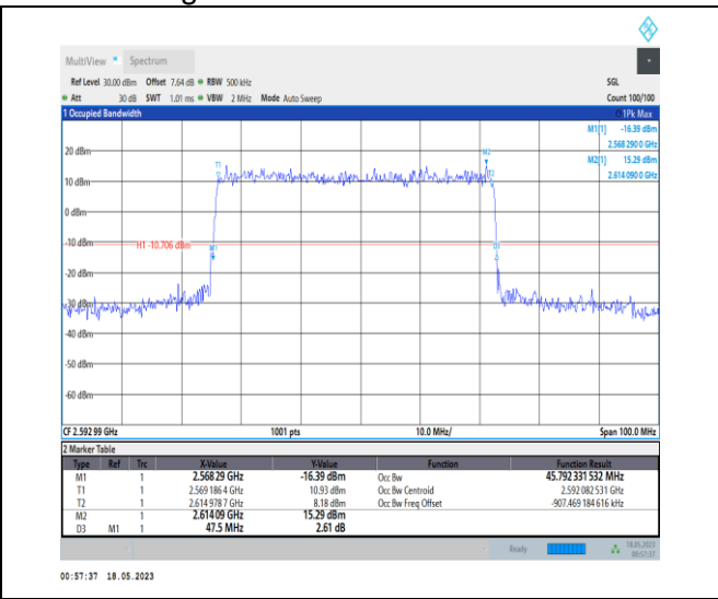
1-N41-PC1-30-50-M-4-DFT-64QAM-Outer_Full-128 @ 0-Ant0-45.792-47.500-≤50-PASS
