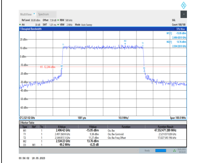
1-N41-PC1-30-50-L-6-CP-QPSK-Outer_Full-133@ 0-Ant0-47.552-49.200-≤50-PASS
