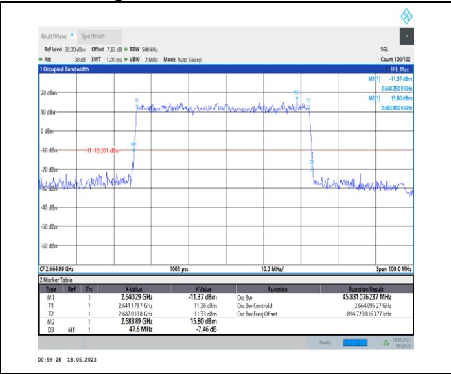
1-N41-PC1-30-50-H-3-DFT-16QAM-Outer_Full-128 @0-Ant0-45.831-47.600-≤50-PASS
