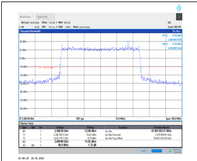
1-N41-PC1-30-50-M-7-CP-16QAM-Outer_Full-133@ 0-Ant0-47.401-49.400-≤50-PASS
