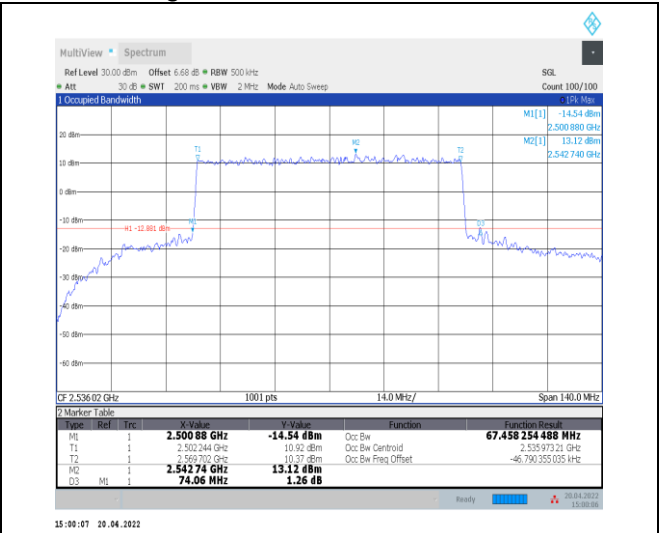
1-N41--30-70-L-7-CP-16QAM-Outer_Full-189@0-Ant0 -67.458-74.060-≤70-PASS
