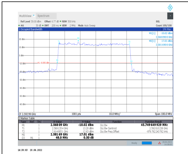
1-N41--30-50-M-3-DFT-16QAM-Outer_Full-128@0-A Ant0-45.75-48.000-≤50-PASS
