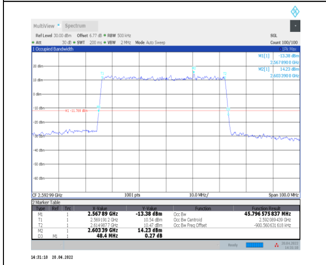
1-N41--30-50-M-5-DFT-256QAM-Outer_Full-128@0-A Ant0-45.797-48.400-≤50-PASS
