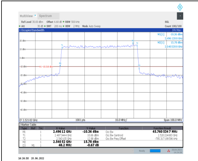
1-N41--30-50-L-4-DFT-64QAM-Outer_Full-128@0-A nt0-45.761-48.200-≤50-PASS
