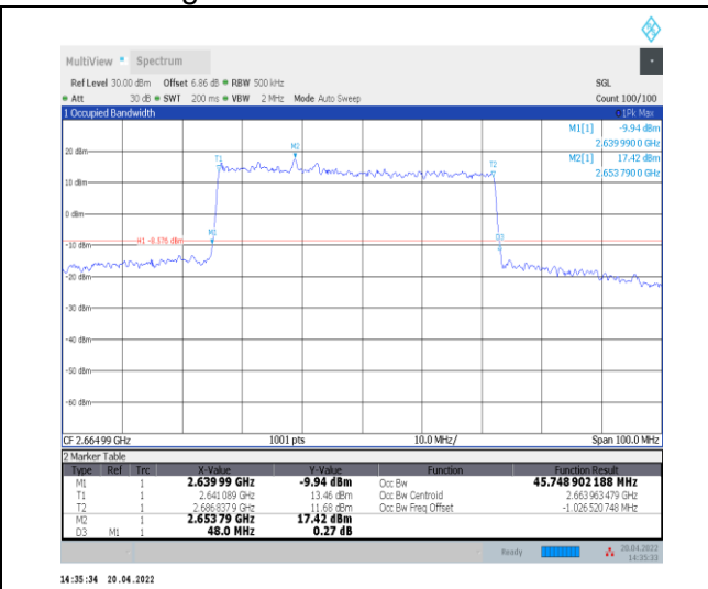
1-N41--30-50-H-3-DFT-16QAM-Outer_Full-128@0-A nt0-45.749-48.000-≤50-PASS
