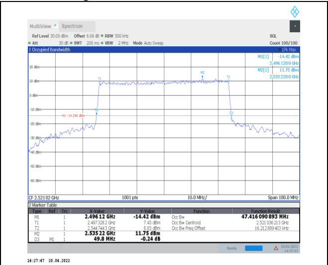
1-N41--30-50-L-9-CP-256QAM-Outer_Full-133@0-A nt0-47.416-49.800-≤50-PASS
