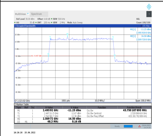
1-N41--30-50-L-3-DFT-16QAM-Outer_Full-128@0-A nt0-45.75-48.300-≤50-PASS
