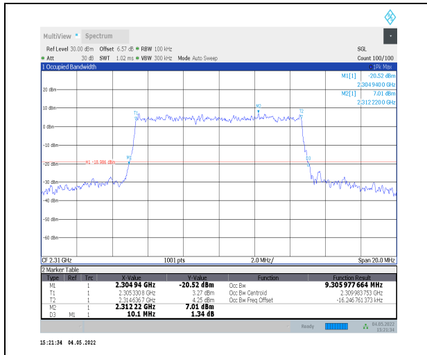
1-N30--15-10-M-9-CP-256QAM-Outer_Full-52@0-A nt0-9.306-10.100-<math>\leq 10</math>-PASS
