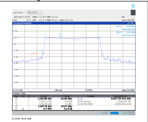
1-N30--15-10-L-3-DFT-16QAM-Outer_Full-50@0-Ant 0-8.958-9.700≤10-PASS
