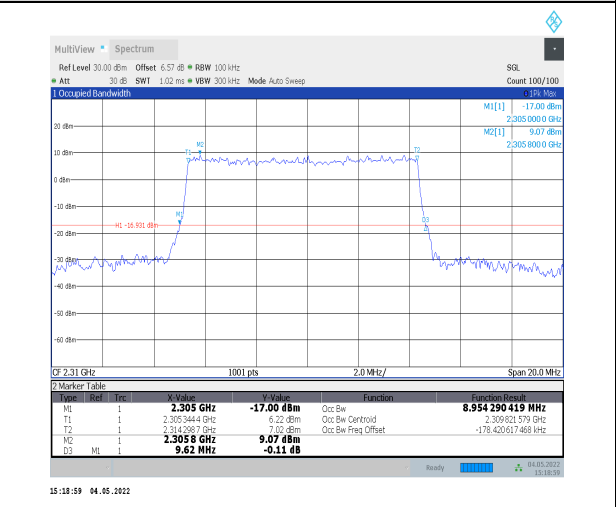
1-N30--15-10-L-5-DFT-256QAM-Outer_Full-50@0-A nt0-8.954-9.620≤10-PASS
