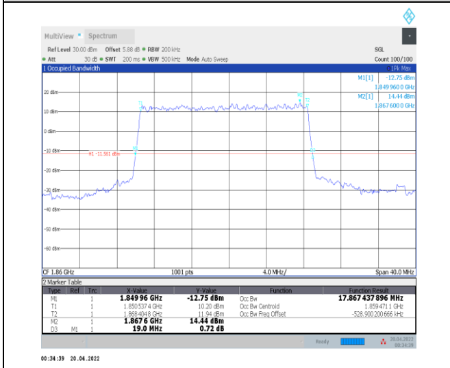
1-N25--15-20-L-2-DFT-PI2BPSK-Outer_Full-100@0-Ant 0-17.867-19.000-≤20-PASS
