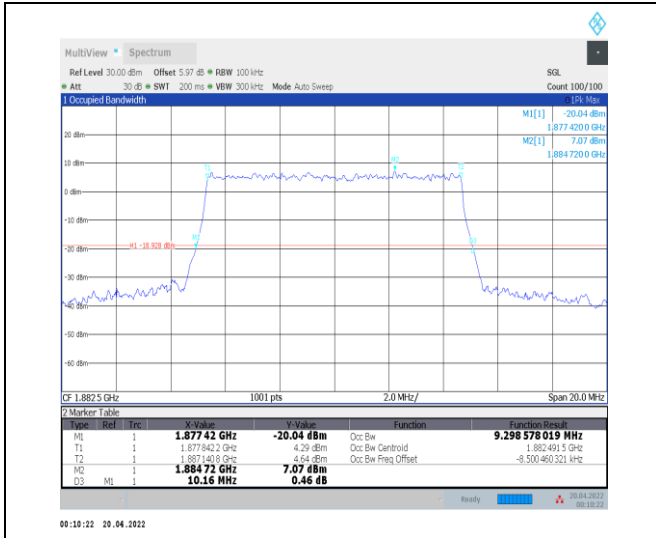
1-N25--15-10-M-9-CP-256QAM-Outer_Full-52@0-A nt0-9.299-10.160-≤10-PASS
