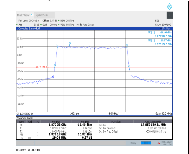
1-N25--15-20-M-4-DFT-64QAM-Outer_Full-100@0-A nt0-17.86-19.080-≤20-PASS
