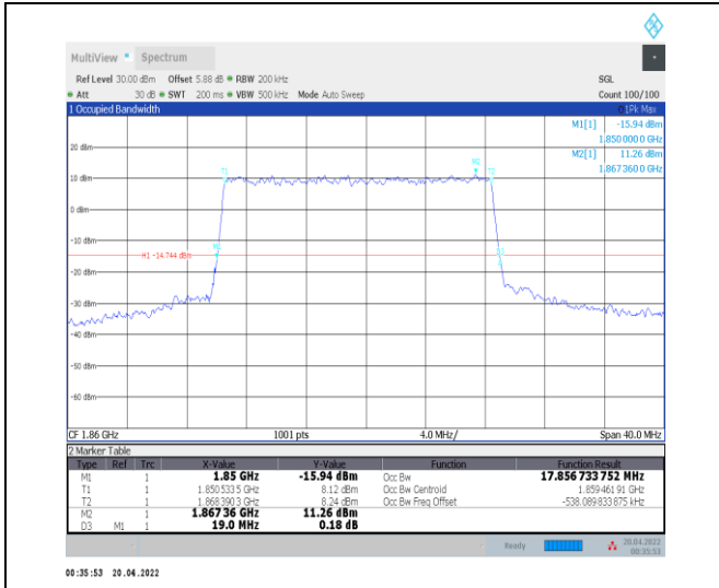
1-N25--15-20-L-4-DFT-64QAM-Outer_Full-100@0-A nt0-17.857-19.000-≤20-PASS
