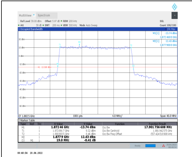
1-N25--15-20-M-3-DFT-16QAM-Outer_Full-100@0-A nt0-17.902-19.000-≤20-PASS
