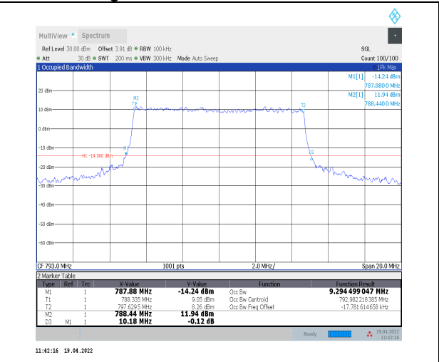
1-N14--15-10-L-7-CP-16QAM-Outer_Full-52@0-Ant0 -9.294-10.180≤10-PASS
