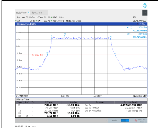
1-N14--15-5-M-2-DFT-PI2BPSK-Outer_Full-25@0-A nt0-4.493-5.160-≤5-PASS
