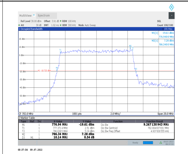
1-N13--15-10-M-9-CP-256QAM-Outer_Full-52@0-Ant0-9.267-10.140-≤10-PASS
