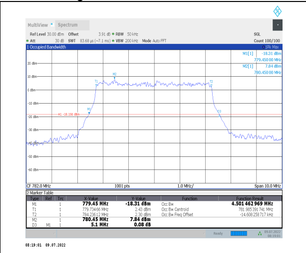
1-N13--15-5-M-9-CP-256QAM-Outer_Full-25@0-Ant 0-4.501-5.100-≤5-PASS
