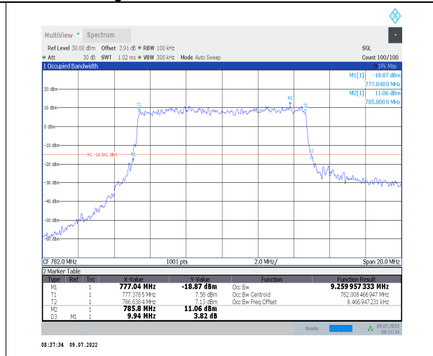
1-N13--15-10-M-7-CP-16QAM-Outer_Full-52@0-Ant0-9.26-9.940-≤10-PASS
