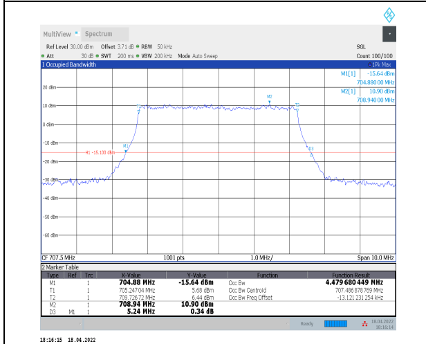
1-N12--15-5-M-6-CP-QPSK-Outer_Full-25@0-Ant0-4 .48-5.240-≤5-PASS
