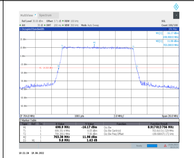
1-N12--15-10-L-5-DFT-256QAM-Outter_Full-50@0-A nt0-8.918-9.800-≤10-PASS
