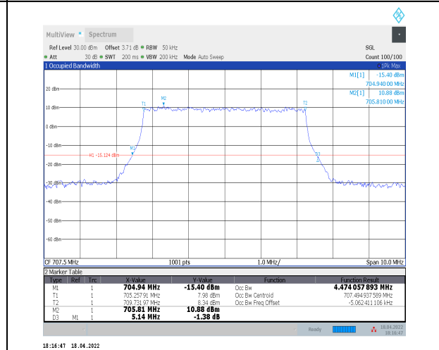
1-N12--15-5-M-7-CP-16QAM-Outer_Full-25@0-Ant0 -4.474-5.140-≤5-PASS
