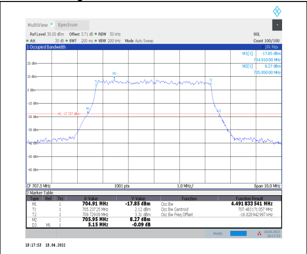
1-N12--15-5-M-9-CP-256QAM-Outer_Full-25@0-Ant 0-4.492-5.150-≤5-PASS
