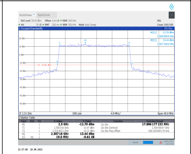
1-N7--15-20-L-3-DFT-16QAM-Outer_Full-100@0-Ant 0-17.886-19.000≤20-PASS
