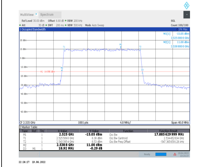
1-N7--15-20-M-5-DFT-256QAM-Outer_Full-100@0-A nt0-17.886-18.920-≤20-PASS
