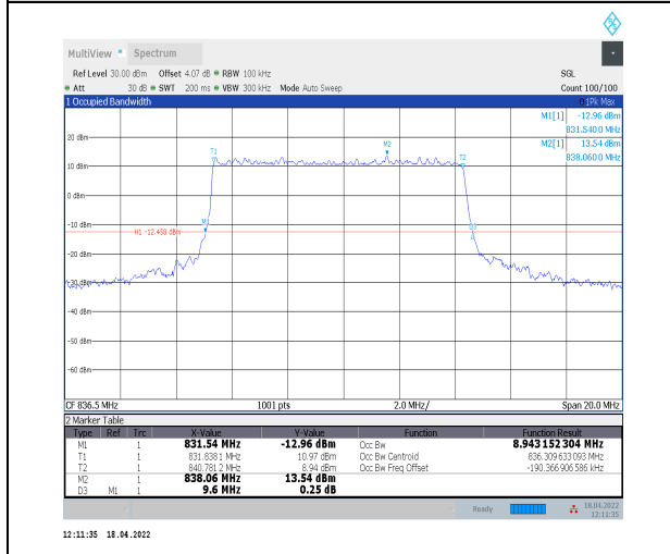
1-N5--15-10-M-3-DFT-16QAM-Outer_Full-50@0-Ant0 0-8.943-9.600-≤10-PASS
