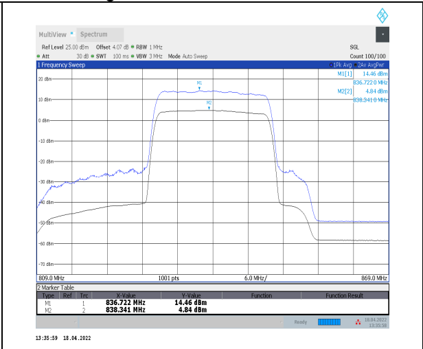
1-N5--15-20-H-2-CP-256QAM-Outer_Full-106@0-A nt0-9.62-100%-0.00-9.62-PASS≤13
