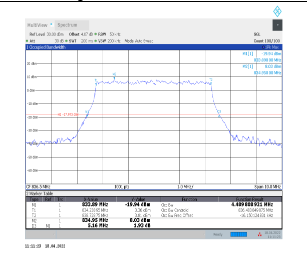
1-N5--15-5-M-9-CP-256QAM-Outer_Full-25@0-Ant0-4.49-5.160-≤5-PASS
