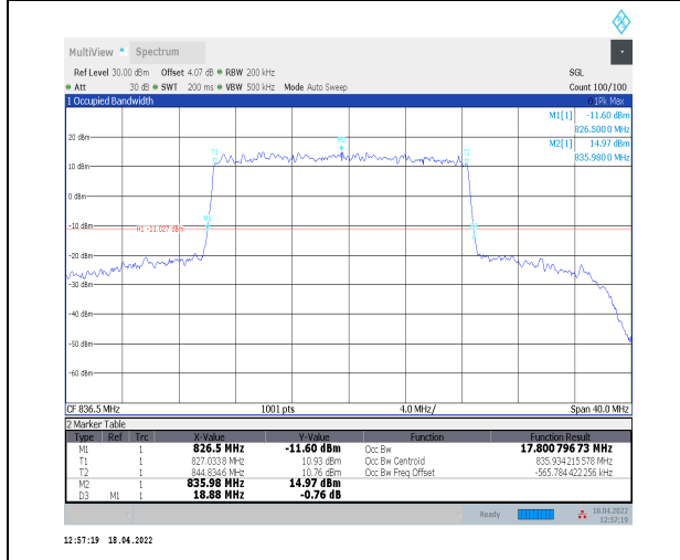
1-N5--15-20-M-1-DFT-QPSK-Outer_Full-100@0-Ant 0-17.801-18.880≤20-PASS
