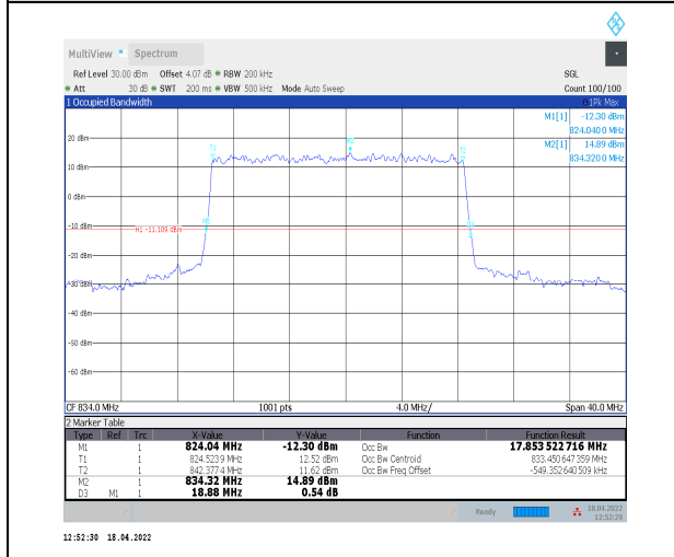
1-N5--15-20-L-2-DFT-PI2BPSK-Outer_Full-100@0-A nt0-17.854-18.880-≤20-PASS
