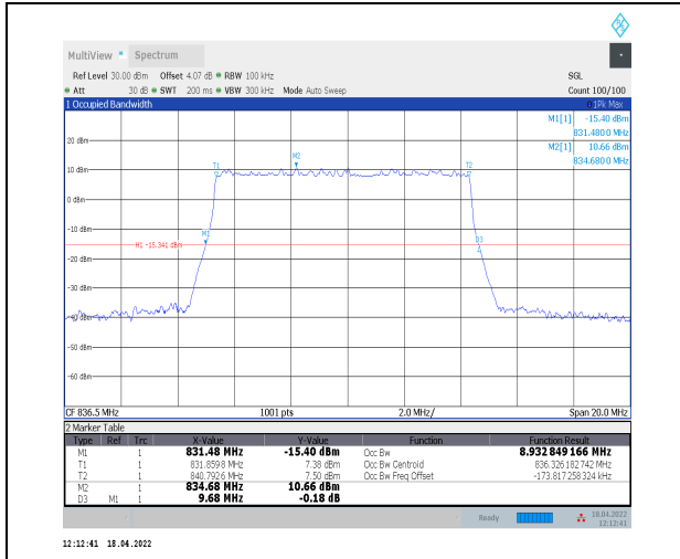
1-N5--15-10-M-5-DFT-256QAM-Outer_Full-50@0-A nt0-8.933-9.680≤10-PASS
