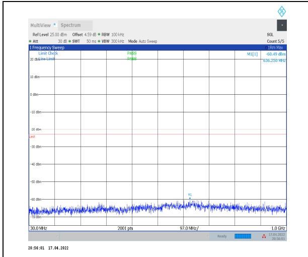
1-N2--15-20-M-1-DFT-PI2BPSK-Inner_1RB_Left-1 @1-30-1000-Ant0--60.49--23-PASS
