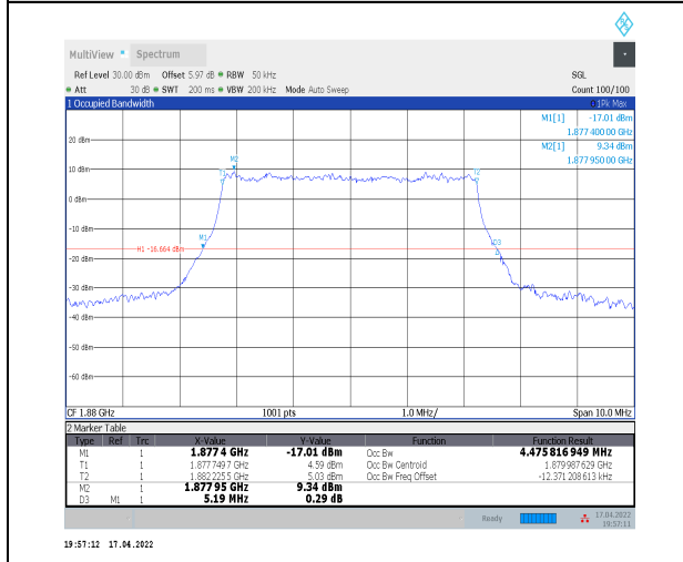
1-N2--15-5-M-6-CP-QPSK-Outer_Full-25@0-Ant0-4. 476-5.190≤5-PASS
