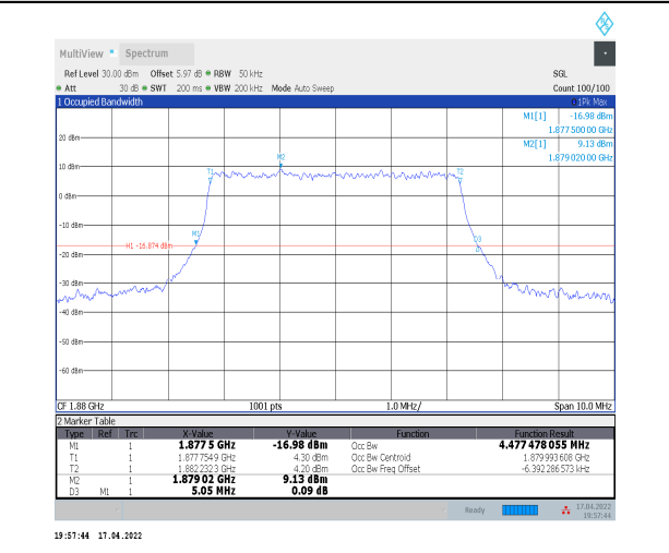
1-N2--15-5-M-7-CP-16QAM-Outer_Full-25@0-Ant0- 4.477-5.050≤5-PASS
