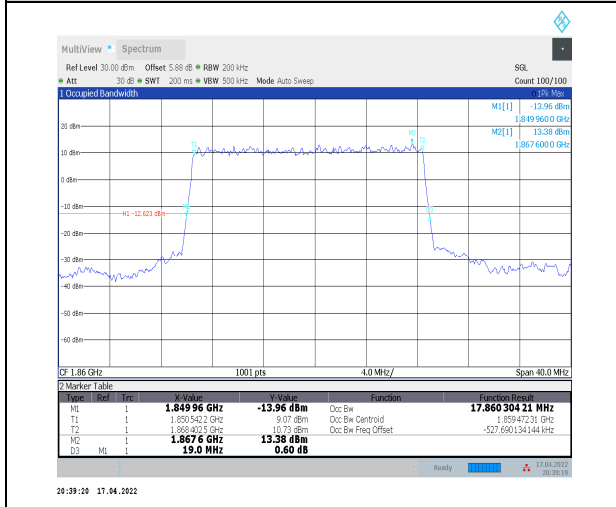
1-N2--15-20-L-2-DFT-PI2BPSK-Outer_Full-100@0-A nt0-17.86-19.000≤20-PASS
