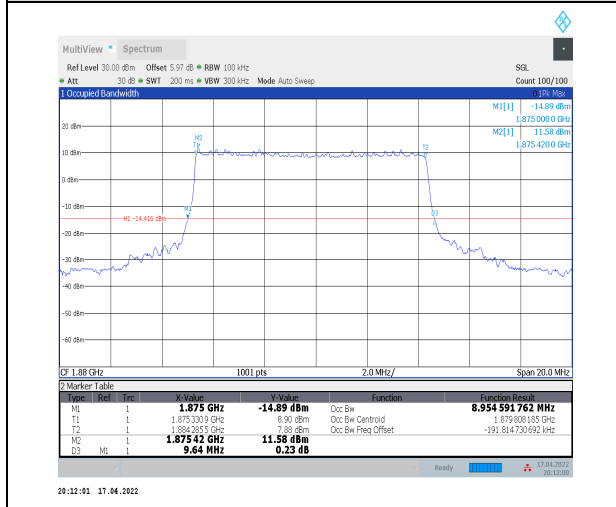
1-N2--15-10-M-3-DFT-16QAM-Outer_Full-50@0-Ant0 0-8.955-9.640-≤10-PASS
