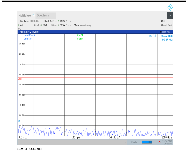
1-N2--15-20-M-1-DFT-PI2BPSK-Inner_1RB_Left-1 @1-0.009-0.15-Ant0--89.02--43-PASS
