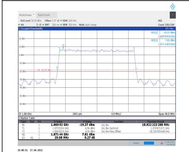
1-N2--15-20-M-9-CP-256QAM-Outer_Full-106@0-A nt0-18.922-20.080-≤20-PASS
