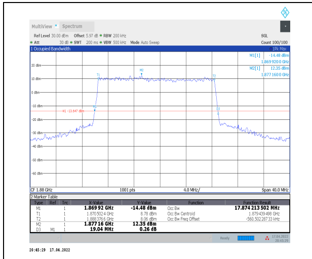
1-N2--15-20-M-3-DFT-16QAM-Outer_Full-100@0-A nt0-17.874-19.040-≤20-PASS
