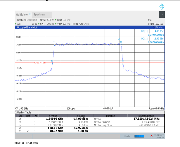
1-N2--15-20-L-1-DFT-QPSK-Outer_Full-100@0-Ant0 -17.85-18.920≤20-PASS
