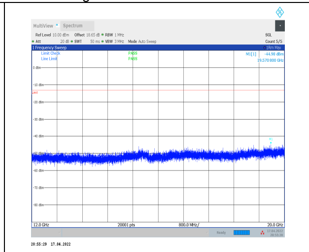
1-N2--15-20-L-1-DFT-PI2BPSK-Inner_1RB_Left-1@1 -12000-20000-Ant0--44.98--13-PASS
