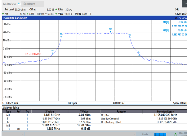
Band25-1.4MHz-QPSK-26365-6RB#0
