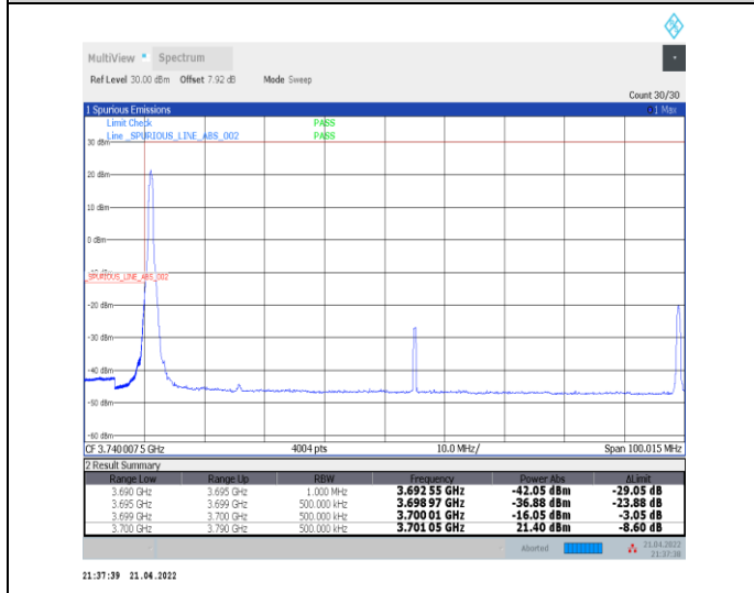
1-N78-3700-3800--30-90-L-4-CP-QPSK-Edge_1RB_L eft-1@0-Ant0-PASS-see graph
