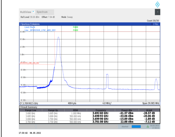
1-N78-3700-3800--30-30-L-4-CP-QPSK-Edge_1RB_L eft-1@0-Ant0-PASS-see graph
