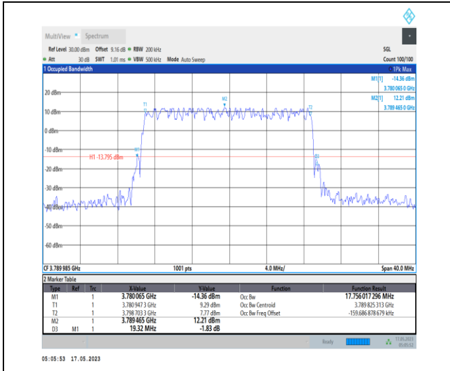
1-N78-3700-3800-PC1-30-20-H-5-DFT-256QAM-Out _Full-50@0-Ant0-17.756-19.320-≤20-PASS
