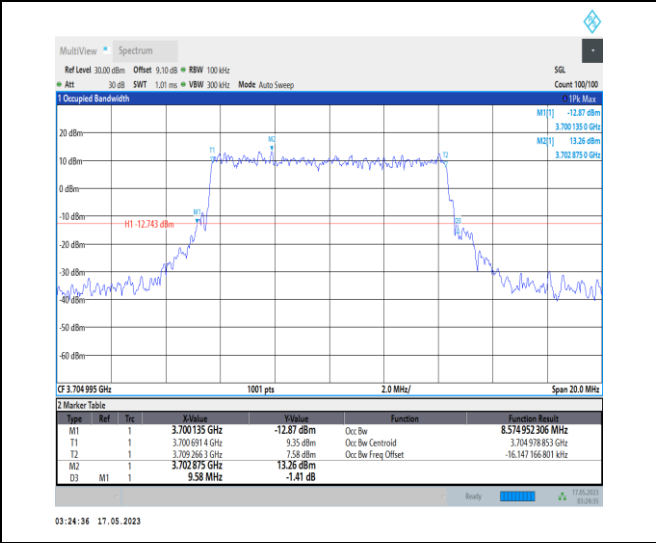
1-N78-3700-3800-PC1-30-10-L-8-CP-64QAM-Outer _Full-24@0-Ant0-8.575-9.580-≤10-PASS
