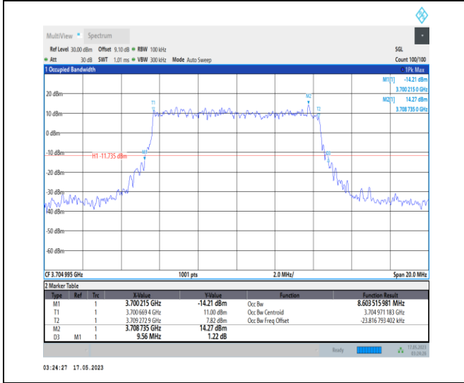
1-N78-3700-3800-PC1-30-10-L-7-CP-16QAM-Outer _Full-24@0-Ant0-8.604-9.560-≤10-PASS
