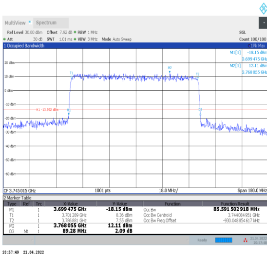
1-N78-3700-3800--30-90-L-4-DFT-64QAM-Outer_Ful l-240@0-Ant0-85.592-89.280-<math>\leq 90</math>-PASS
