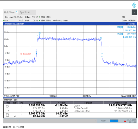
1-N78-3700-3800--30-90-L-3-DFT-16QAM-Outer_Fu ll-240@0-Ant0-85.615-88.740-<math>\leq 90</math>-PASS
