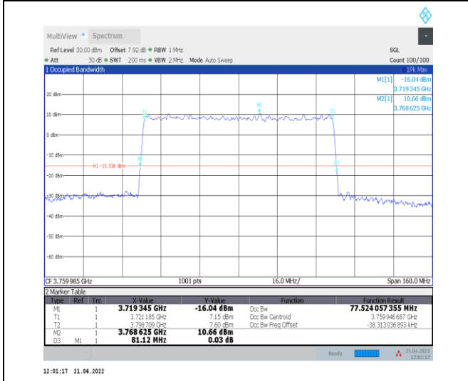
1-N78-3700-3800--30-80-H-9-CP-256QAM-Outer_Fu ll-217@0-Ant0-77.524-81.120-<math>\leq 80</math>-PASS
