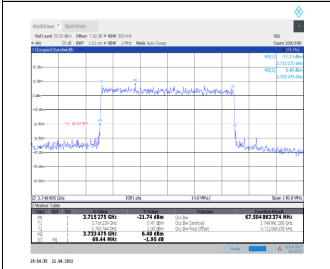
1-N78-3700-3800--30-70-M-9-CP-256QAM-Outer_F ull-189@0-Ant0-67.505-69.440-≤70-PASS
