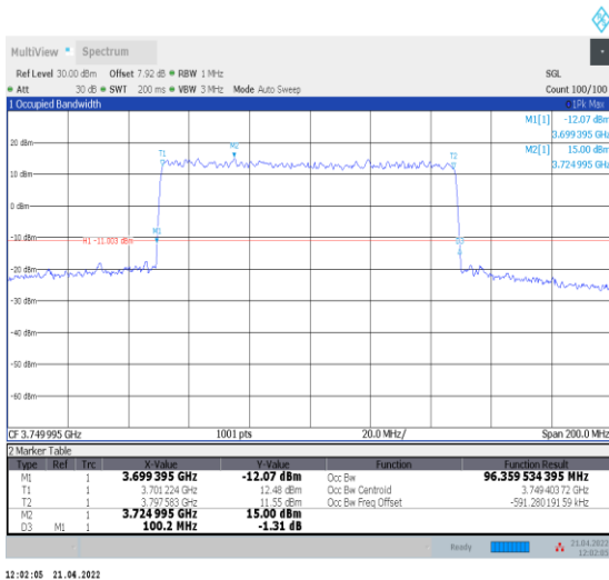
1-N78-3700-3800--30-100-L-1-DFT-QPSK-Outer_Full I-270@0-Ant0-96.36-100.200-≤100-PASS
