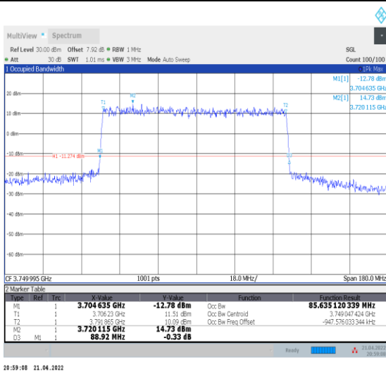
1-N78-3700-3800--30-90-M-1-DFT-QPSK-Outer_Full -240@0-Ant0-85.635-88.920-≤90-PASS
