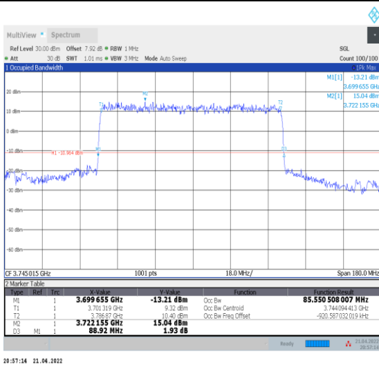
1-N78-3700-3800--30-90-L-2-DFT-PI2BPSK-Outer_F ull-240@0-Ant0-85.551-88.920-<math>\leq 90</math>-PASS
