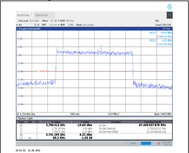
1-N78-3700-3800--30-70-L-9-CP-256QAM-Outer_Fu II-189@0-Ant0-67.47-69.300-≤70-PASS
