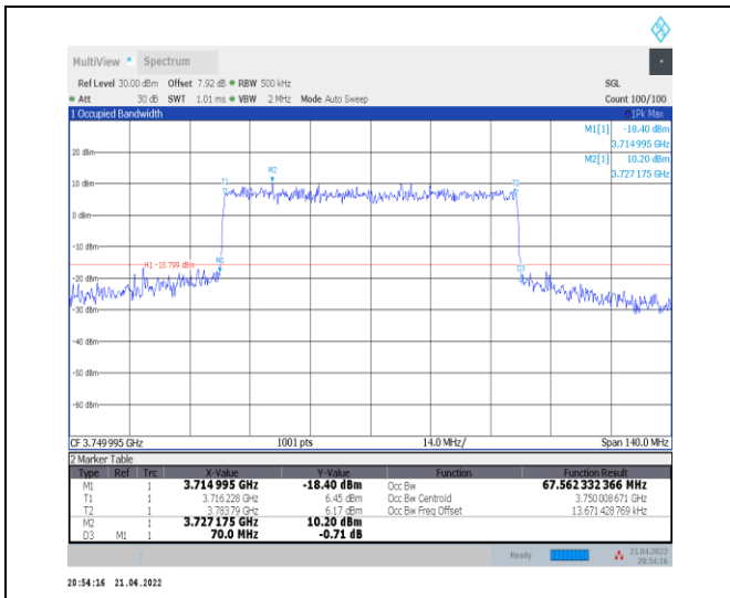
1-N78-3700-3800--30-70-M-7-CP-16QAM-Outer_Full -189@0-Ant0-67.562-70.000-≤70-PASS
