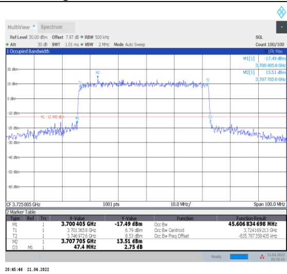
1-N78-3700-3800--30-50-L-3-DFT-16QAM-Outer_Fu ll-128@0-Ant0-45.607-47.400-≤50-PASS
