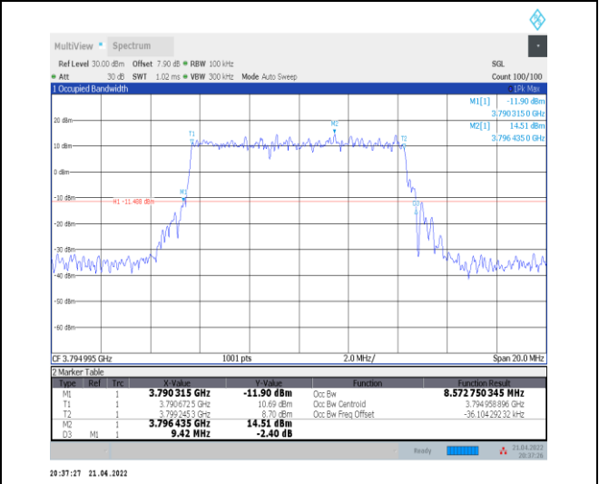
1-N78-3700-3800--30-10-H-2-DFT-PI2BPSK-Outer_Full-24@0-Ant0-8.573-9.420-≤10-PASS
