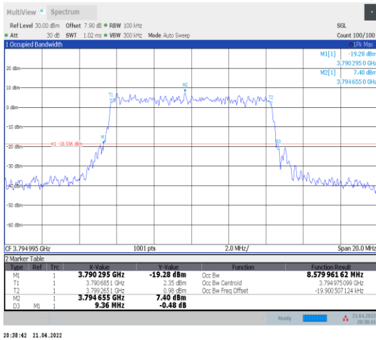
1-N78-3700-3800--30-10-H-9-CP-256QAM-Outer_Fu ll-24@0-Ant0-8.58-9.360≤10-PASS
