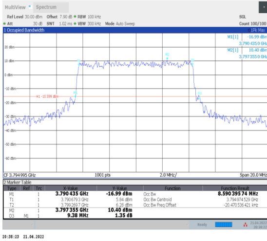
1-N78-3700-3800--30-10-H-7-CP-16QAM-Outer_Full -24@0-Ant0-8.59-9.380≤10-PASS
