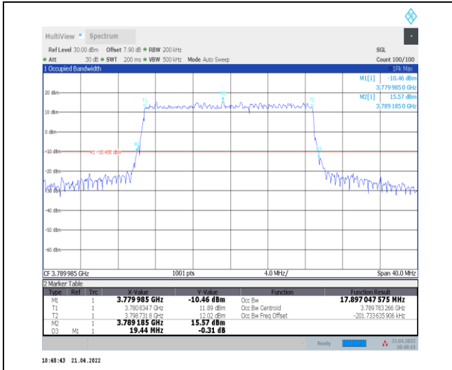
1-N78-3700-3800--30-20-H-1-DFT-QPSK-Outer_Full -50@0-Ant0-17.897-19.440-≤20-PASS
