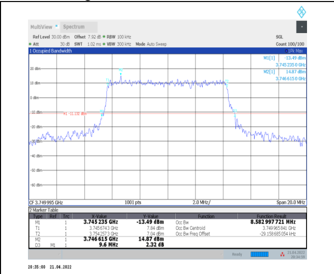
1-N78-3700-3800--30-10-M-1-DFT-QPSK-Outer_Full -24@0-Ant0-8.583-9.600-≤10-PASS
