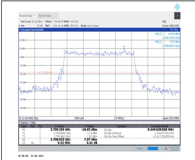
1-N78-3700-3800--30-10-L-9-CP-256QAM-Outer_Fu II-24@0-Ant0-8.55-9.320-≤10-PASS
