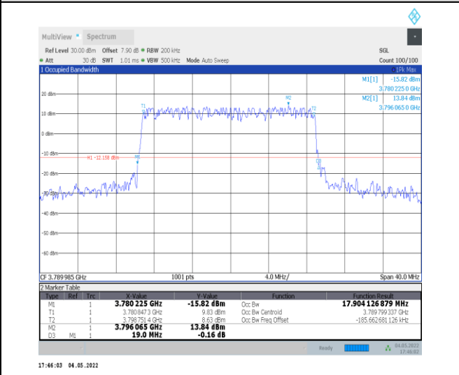
1-N78-3700-3800--30-20-H-4-DFT-64QAM-Outer_Fu II-50@0-Ant0-17.904-19.000-≤20-PASS
