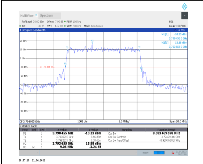
1-N78-3700-3800--30-10-H-1-DFT-QPSK-Outer_Full -24@0-Ant0-8.583-9.060-≤10-PASS
