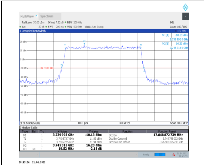
1-N78-3700-3800--30-20-M-2-DFT-PI2BPSK-Outer_Full-50@0-Ant0-17.849-19.520-≤20-PASS
