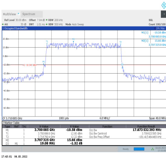
1-N78-3700-3800--30-20-L-1-DFT-QPSK-Outer_Full -50@0-Ant0-17.874-19.080-≤20-PASS
