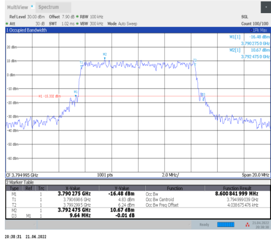
1-N78-3700-3800--30-10-H-8-CP-64QAM-Outer_Full -24@0-Ant0-8.601-9.640≤10-PASS
