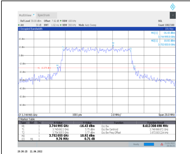
1-N78-3700-3800--30-10-M-8-CP-64QAM-Outer_Full -24@0-Ant0-8.613-9.760-≤10-PASS
