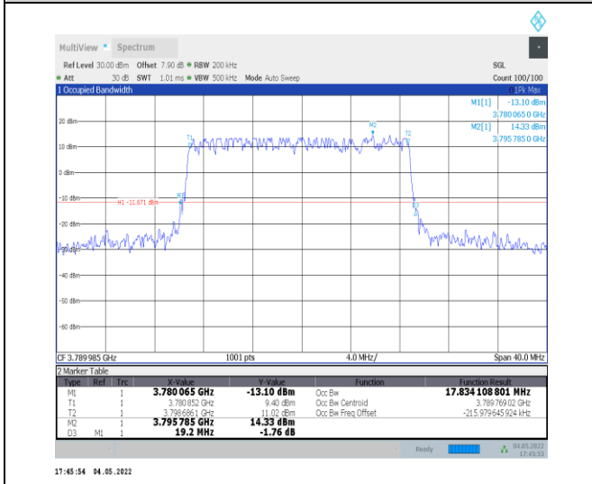
1-N78-3700-3800--30-20-H-3-DFT-16QAM-Outer_Fu II-50@0-Ant0-17.834-19.200-≤20-PASS
