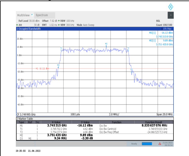
1-N78-3700-3800--30-10-M-5-DFT-256QAM-Outer_Full-24@0-Ant0-8.536-9.340-≤10-PASS
