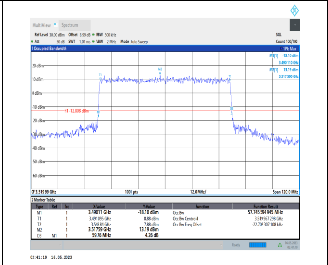
1-N78-3450-3550-PC1-30-60-H-8-CP-64QAM-Outer _Full-162@0-Ant0-57.746-59.760-≤60-PASS
