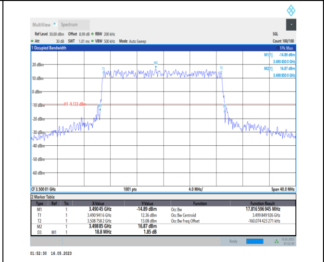
1-N78-3450-3550-PC1-30-20-M-1-DFT-QPSK-Outer_Full-50@0-Ant0-17.817-18.800-≤20-PASS
