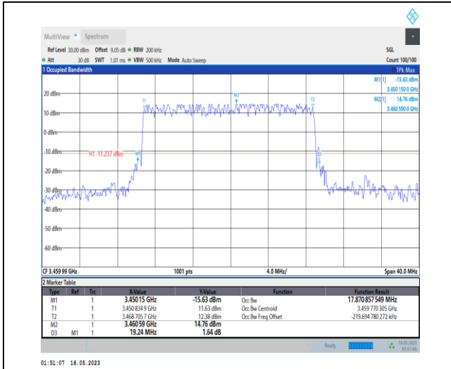
1-N78-3450-3550-PC1-30-20-L-3-DFT-16QAM-Outer_Full-50@0-Ant0-17.871-19.240-≤20-PASS
