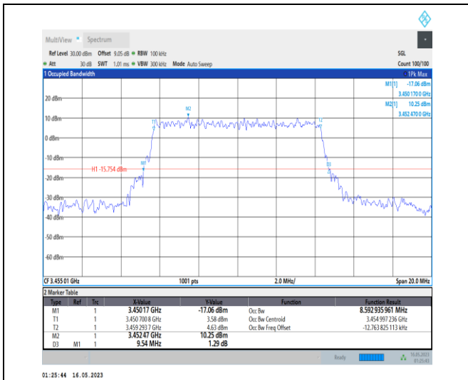
1-N78-3450-3550-PC1-30-10-L-9-CP-256QAM-Outer_Full-24@0-Ant0-8.593-9.540-≤10-PASS
