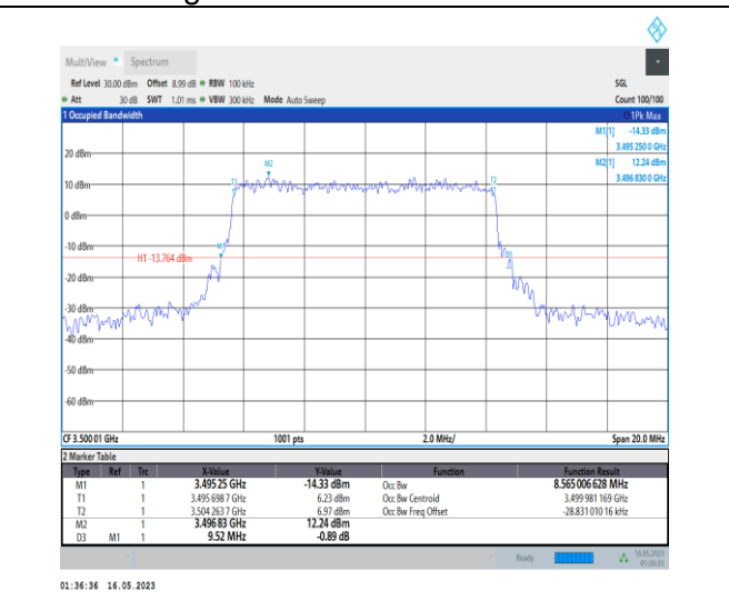
1-N78-3450-3550-PC1-30-10-M-5-DFT-256QAM-Out er_Full-24@0-Ant0-8.565-9.520-≤10-PASS
