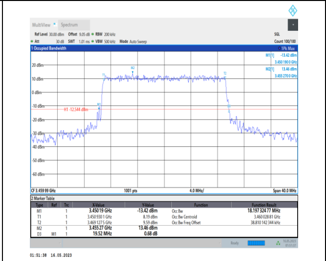
1-N78-3450-3550-PC1-30-20-L-6-CP-QPSK-Outer_Full-51@0-Ant0-18.197-19.520-≤20-PASS
