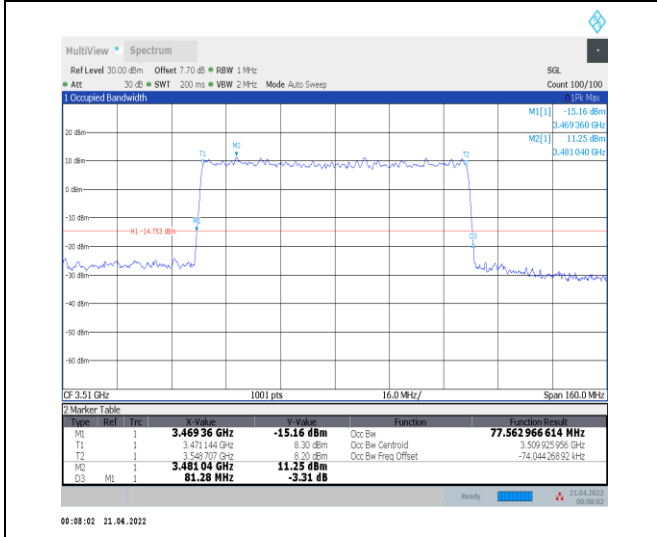
1-N78-3450-3550--30-80-H-9-CP-256QAM-Outer_Fu II-217@0-Ant0-77.563-81.280-≤80-PASS
