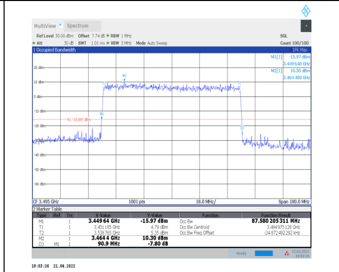
1-N78-3450-3550--30-90-L-9-CP-256QAM-Outer_Fu II-245@0-Ant0-87.58-90.900<=90-PASS
