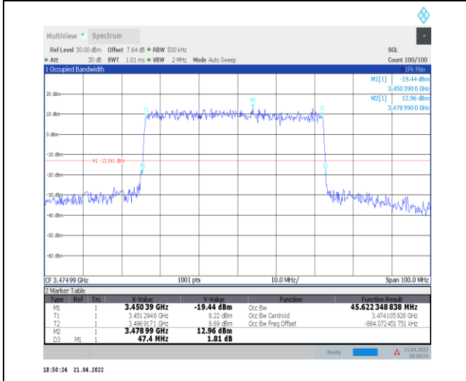
1-N78-3450-3550--30-50-L-4-DFT-64QAM-Outer_Ful l-128@0-Ant0-45.622-47.400-≤50-PASS
