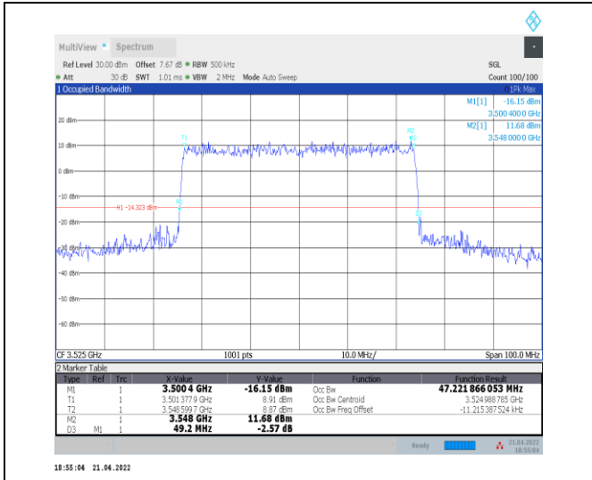
1-N78-3450-3550--30-50-H-8-CP-64QAM-Outer_Full -133@0-Ant0-47.222-49.200-≤50-PASS
