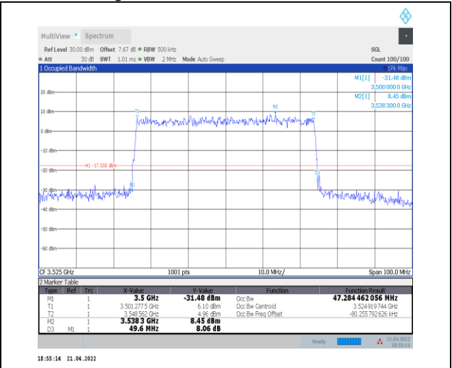
1-N78-3450-3550--30-50-H-9-CP-256QAM-Outer_Full -133@0-Ant0-47.284-49.600-≤50-PASS
