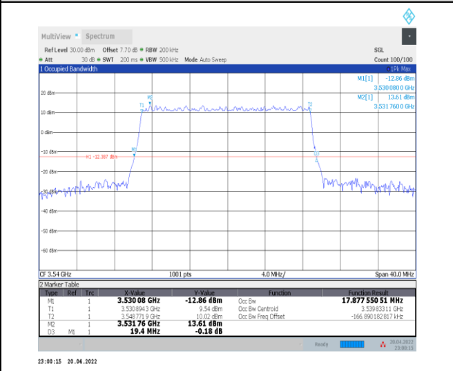
1-N78-3450-3550--30-20-H-4-DFT-64QAM-Outer_Fu II-50@0-Ant0-17.878-19.400-≤20-PASS
