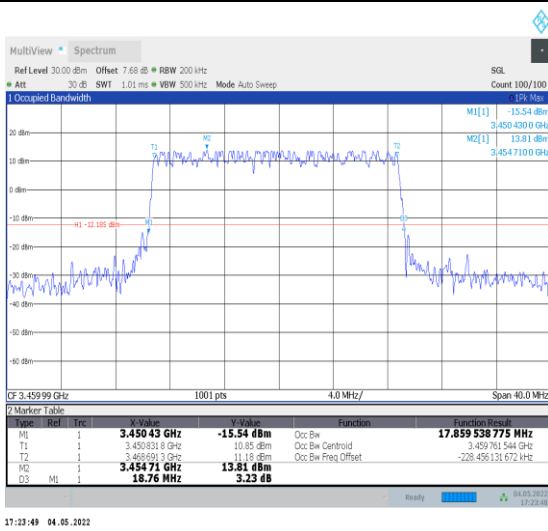
1-N78-3450-3550--30-20-L-3-DFT-16QAM-Outer_Ful I-50@0-Ant0-17.86-18.760-<=20-PASS
