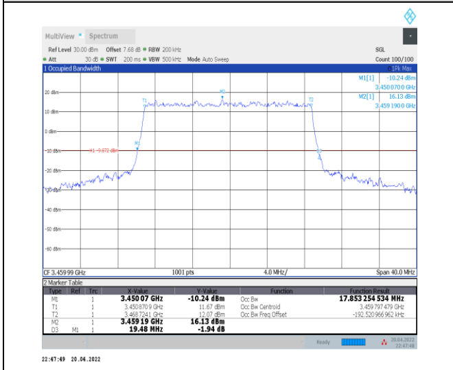
1-N78-3450-3550--30-20-L-1-DFT-QPSK-Outer_Full -50@0-Ant0-17.853-19.480-≤20-PASS
