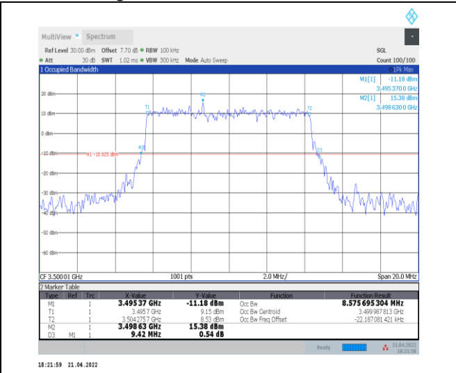
1-N78-3450-3550--30-10-M-1-DFT-QPSK-Outer_Full -24@0-Ant0-8.576-9.420-≤10-PASS
