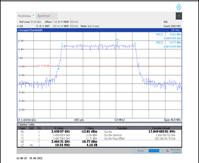
1-N78-3450-3550--30-20-L-2-DFT-PI2BPSK-Outer_Full -50@0-Ant0-17.85-19.440-≤20-PASS
