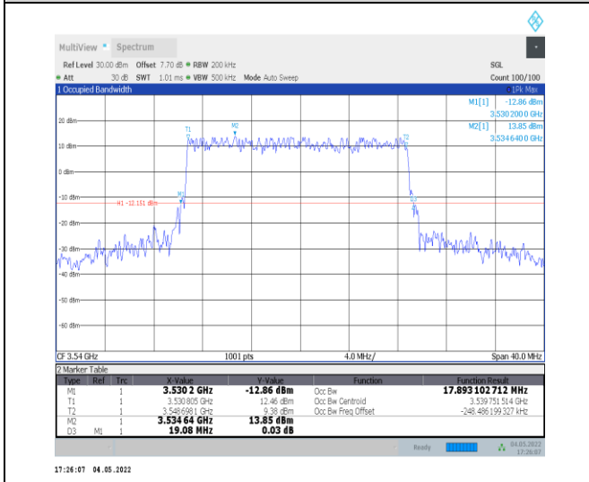
1-N78-3450-3550--30-20-H-3-DFT-16QAM-Outer_Fu II-50@0-Ant0-17.893-19.080-≤20-PASS
