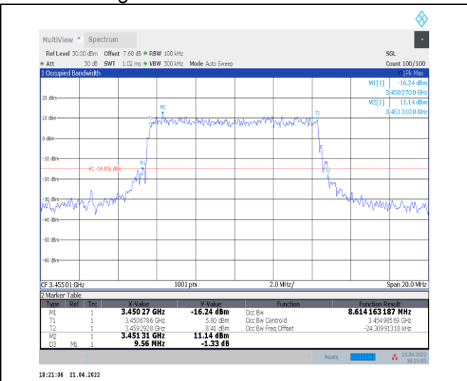
1-N78-3450-3550--30-10-L-6-CP-QPSK-Outer_Full-24@0-Ant0-8.614-9.560-≤10-PASS
