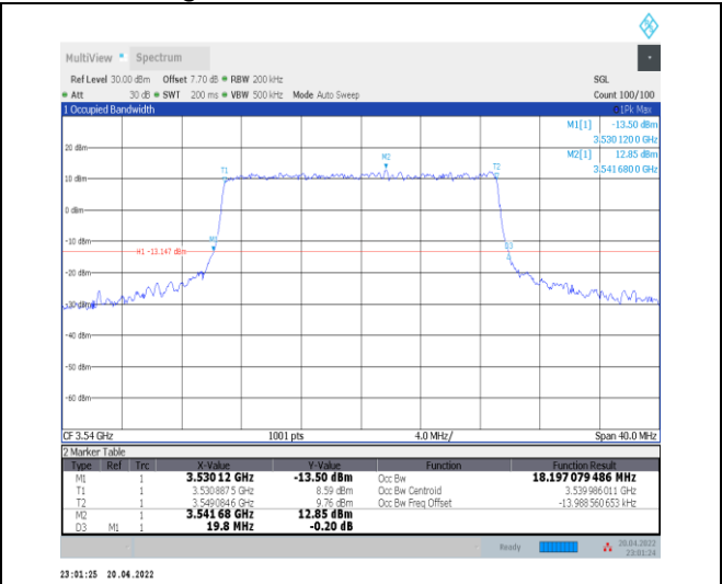
1-N78-3450-3550--30-20-H-6-CP-QPSK-Outer_Full-51@0-Ant0-18.197-19.800-≤20-PASS
