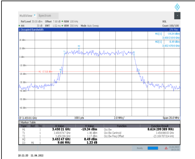
1-N78-3450-3550--30-10-L-9-CP-256QAM-Outer_Fu II-24@0-Ant0-8.624-9.660-≤10-PASS
