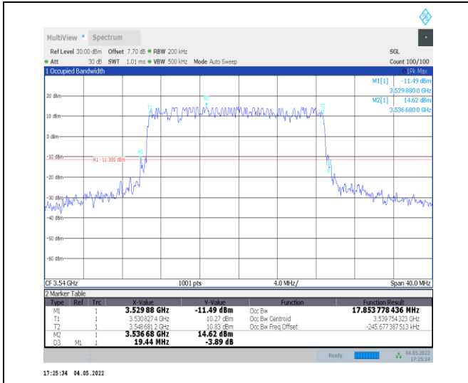
1-N78-3450-3550--30-20-H-1-DFT-QPSK-Outer_Full -50@0-Ant0-17.854-19.440-≤20-PASS
