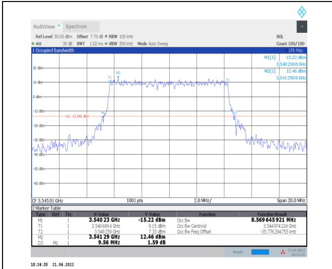
1-N78-3450-3550--30-10-H-3-DFT-16QAM-Outer_Fu II-24@0-Ant0-8.57-9.560-≤10-PASS
