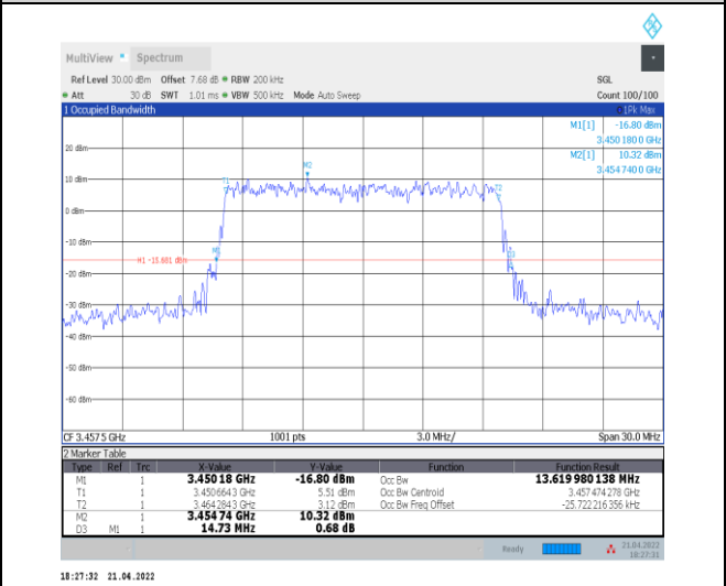
1-N78-3450-3550--30-15-L-9-CP-256QAM-Outer_Fu ll-38@0-Ant0-13.62-14.730-≤15-PASS
