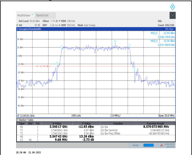
1-N78-3450-3550--30-10-H-4-DFT-64QAM-Outer_Fu II-24@0-Ant0-8.57-9.680-≤10-PASS
