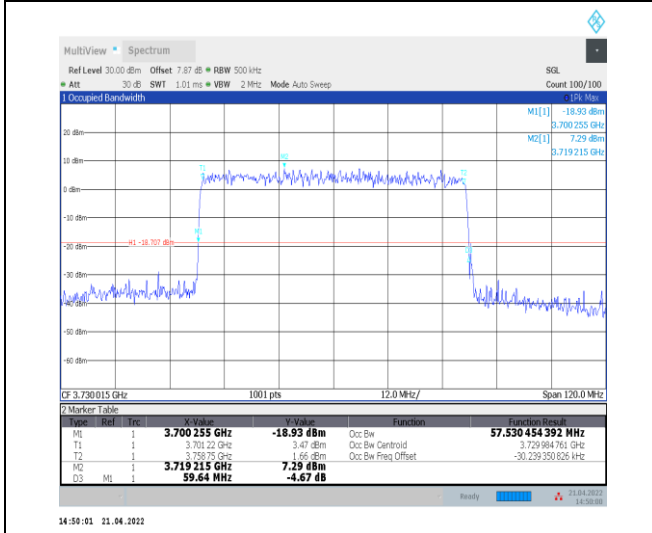
1-N77-3700-3980--30-60-L-9-CP-256QAM-Outer_Fu ll-162@0-Ant0-57.53-59.640-≤60-PASS
