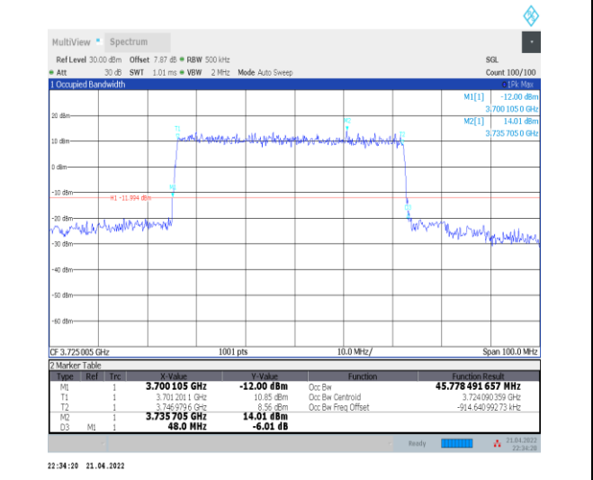
1-N77-3700-3980--30-50-L-1-DFT-QPSK-Outer_Full -128@0-Ant0-45.778-48.000≤50-PASS
