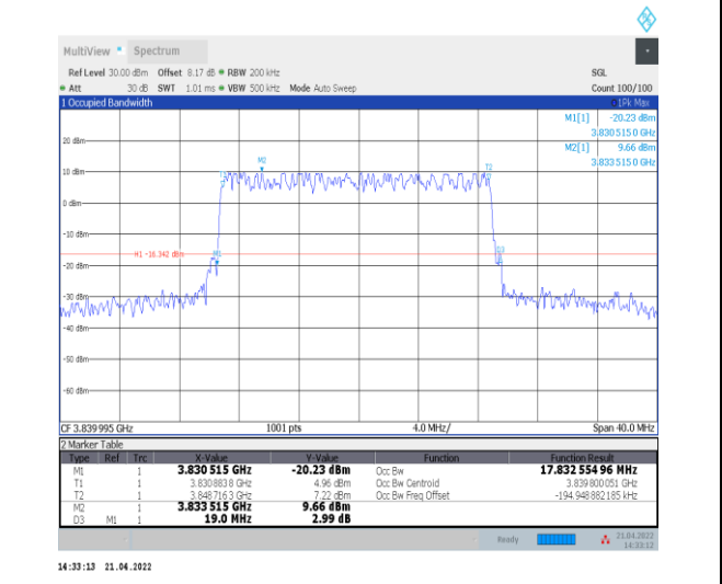
1-N77-3700-3980--30-20-M-5-DFT-256QAM-Outer_Full-50@0-Ant0-17.833-19.000-≤20-PASS
