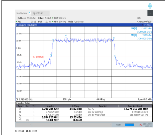
1-N77-3700-3980--30-20-L-1-DFT-QPSK-Outer_Full -50@0-Ant0-17.775-18.840≤20-PASS
