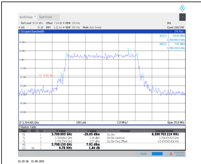
1-N77-3700-3980--30-10-L-9-CP-256QAM-Outer_Fu ll-24@0-Ant0-8.591-9.780-<=10-PASS
