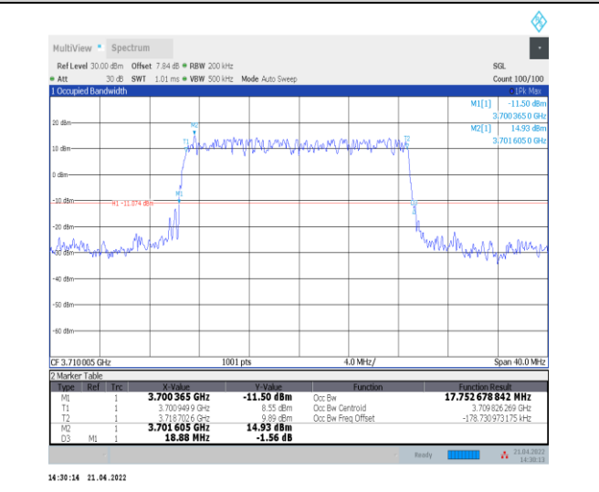
1-N77-3700-3980--30-20-L-2-DFT-PI2BPSK-Outer_Full -50@0-Ant0-17.753-18.880≤20-PASS
