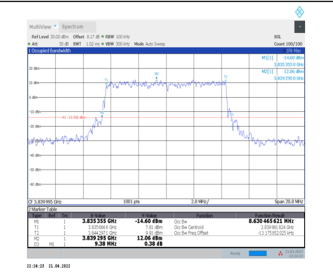
1-N77-3700-3980--30-10-M-3-DFT-16QAM-Outer_Fu ll-24@0-Ant0-8.63-9.380-<=10-PASS
