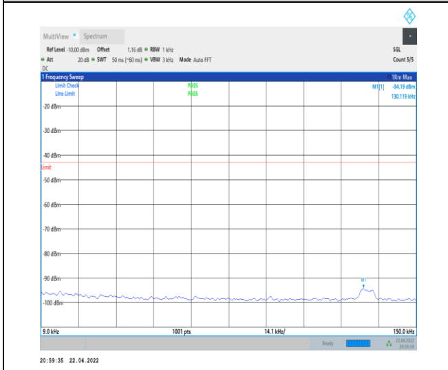
1-N66-PC3-15-40-M-1-DFT-PI2BPSK-Inner_1RB_L eft-1@1-0.009-0.15-Ant0--94.19--43-PASS
