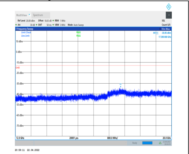
1-N66-PC3-15-40-L-1-DFT-PI2BPSK-Inner_1RB_Lef t-1@1-12000-20000-Ant0--33.95--13-PASS
