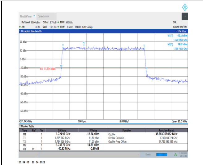
1-N66-PC3-15-40-M-1-DFT-QPSK-Outer_Full-216@ 0-Ant0-38.584-40.320-≤40-PASS
